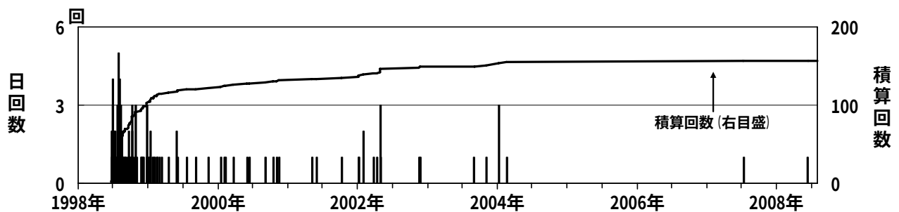
図 3※ 岩手山 日別微動回数（1998 年 1 月～2008 年 7 月）
