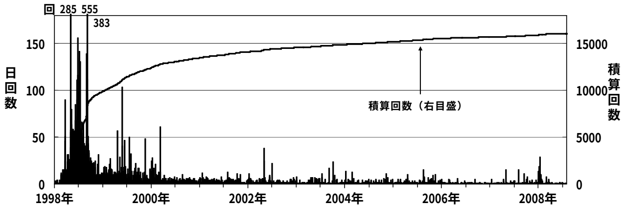
図 2※ 岩手山 日別地震回数（1998 年 1 月～2008 年 7 月）
