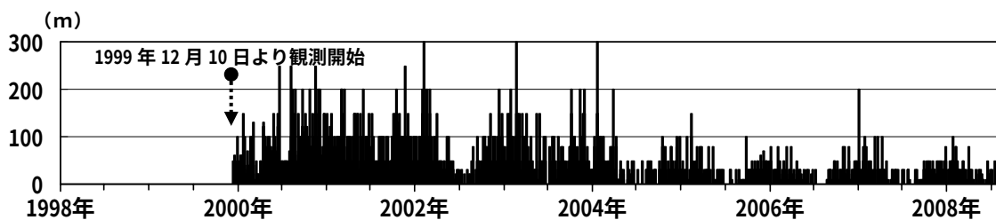
図 4 岩手山 日最大噴気の高さ（黒倉山）（1999 年 12 月 10 日～2008 年 7 月）
