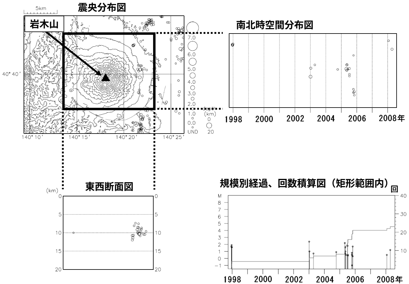
図 2 ※ 岩木山周辺の地震活動（1997 年 10 月～2008 年 7 月）
