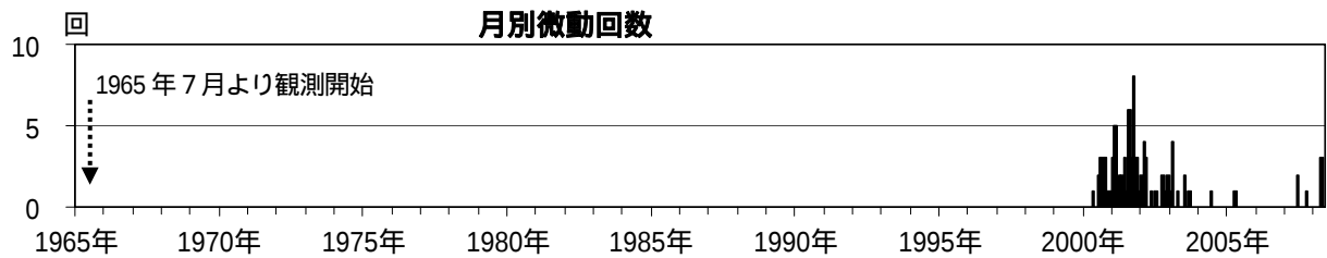
図3 磐梯山 月別地震回数、月別微動回数(1965 年 7 月～2008 年 5 月)
