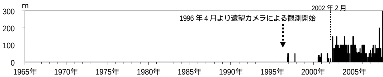
図2 磐梯山 月最大噴気高（1996 年 4 月～2008 年 5 月）
