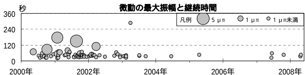
図4 磐梯山 日別地震回数、日別微動回数、微動の振幅と継続時間 (2000 年 1 月～2008 年 5 月)
