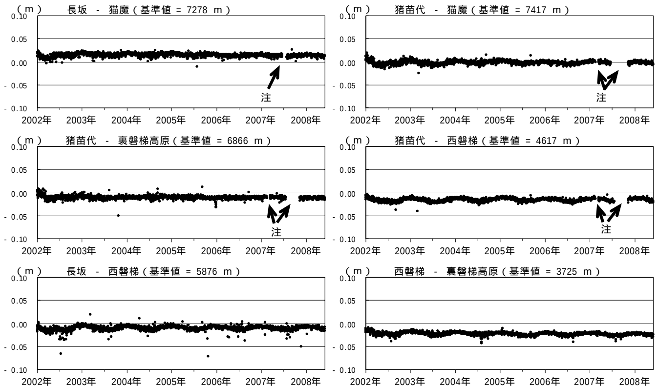
図6 磐梯山 GPS 基線長変化図（2002 年 1 月～2008 年 5 月）
