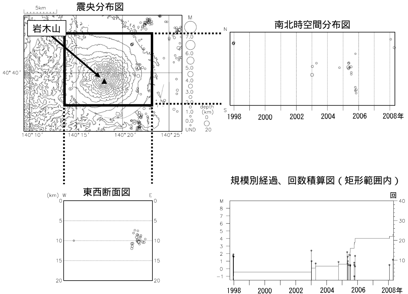
図 2 岩木山周辺の地震活動（1997 年 10 月～2008 年 4 月）
