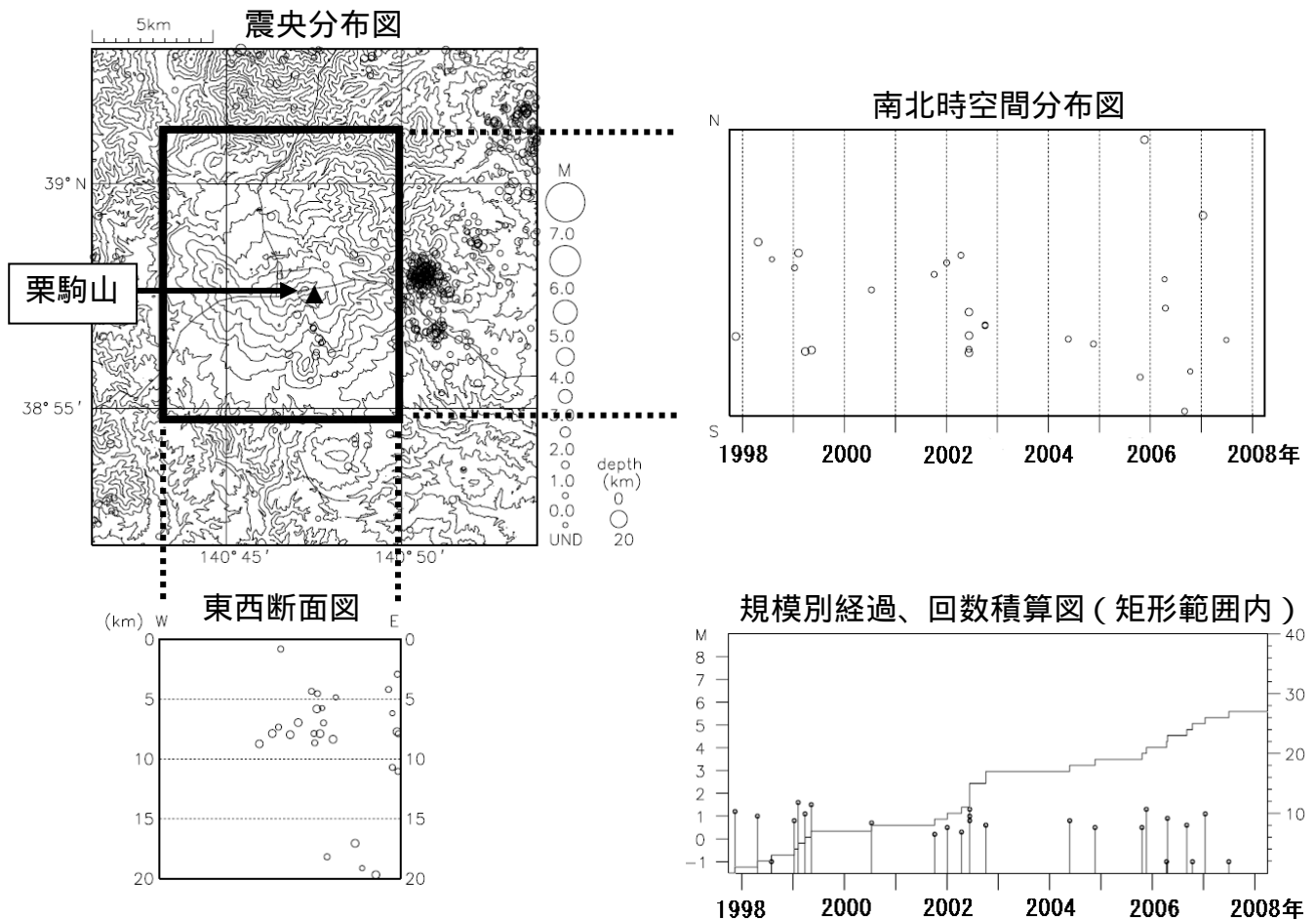
図 3 栗駒山周辺の地震活動（1997 年 10 月～2008 年 3 月）
