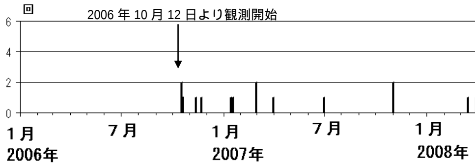
図 2 栗駒山 日別地震回数（2006 年 10 月～2008 年 3 月）
