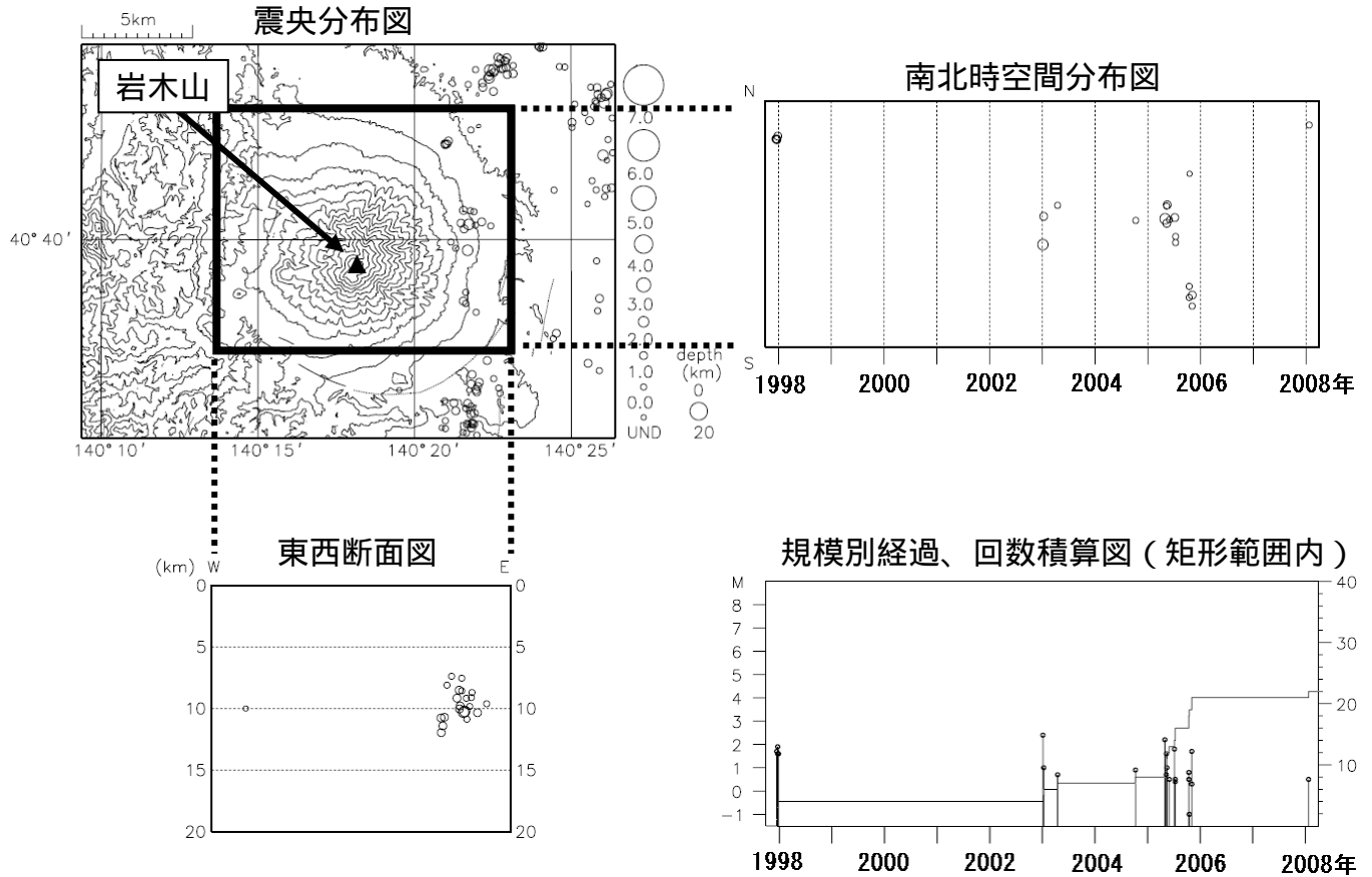
図 2 岩木山周辺の地震活動（1997 年 10 月～2008 年 3 月）
