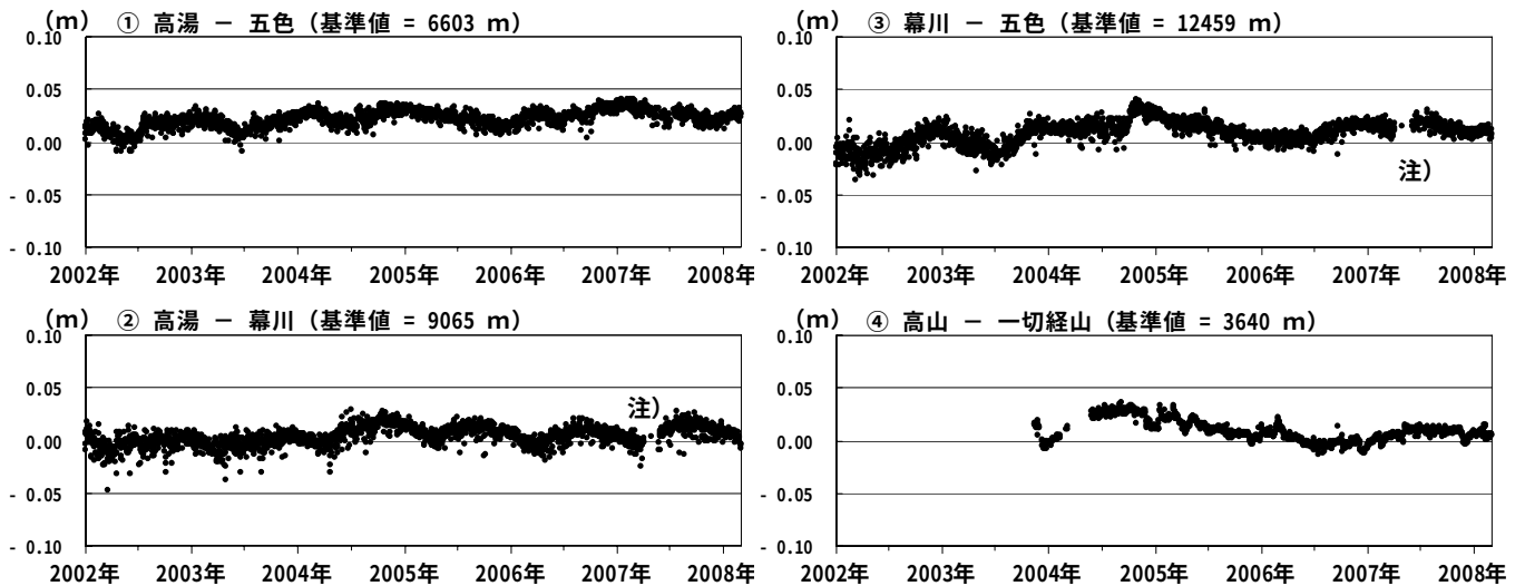
図 5 吾妻山 GPS 基線長変化図（2002 年 1 月～2008 年 2 月）
