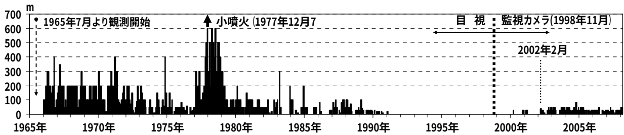
図2 吾妻山 月別最大噴気（噴煙）高（1965 年 7 月～2008 年 2 月）
