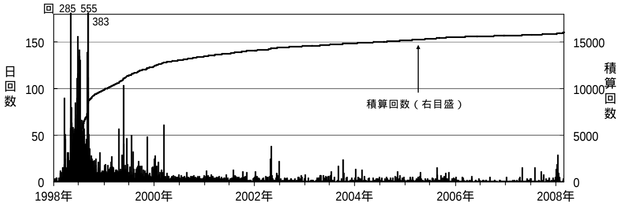
図 2 岩手山 日別地震回数（1998 年 1 月～2008 年 2 月）
