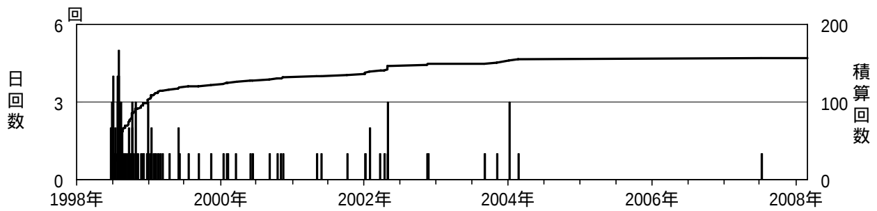
図 3 岩手山 日別微動回数（1998 年 1 月～2008 年 2 月）
