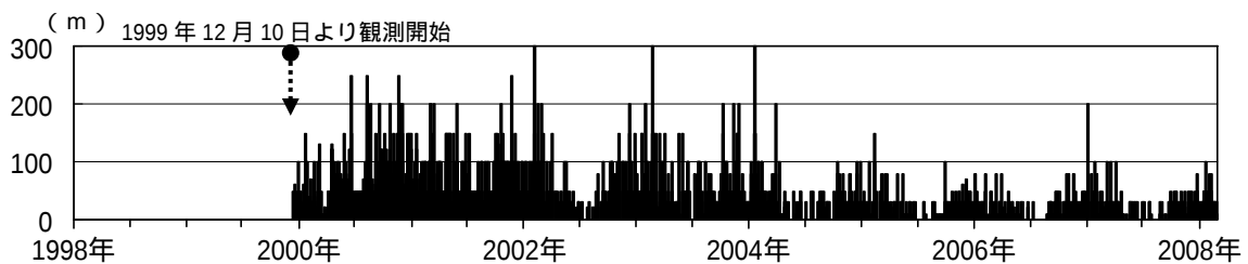
図 4 岩手山 日最大噴気の高さ（黒倉山）（1999 年 12 月 10 日～2008 年 2 月）
