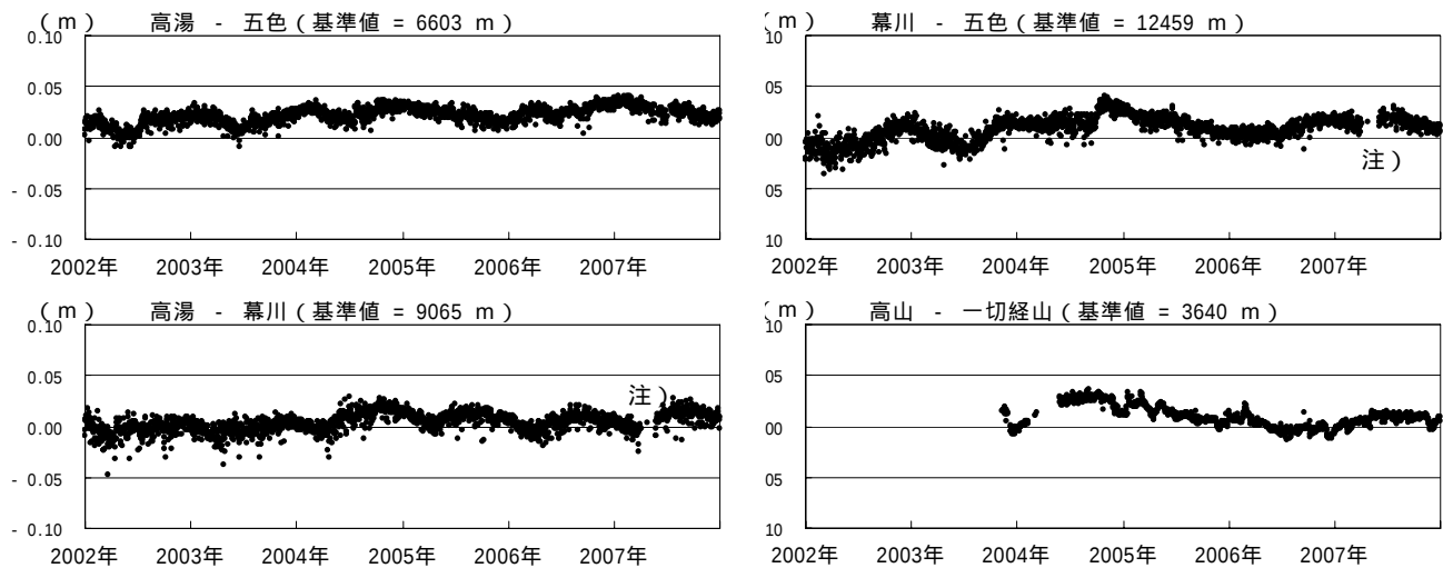
図 5 吾妻山 GPS 基線長変化図（2002 年 1 月～2007 年 12 月） ～ は図 4 の GPS 基線 ～ に対応しています。 注）幕川観測点障害のため、一部に欠測があります。
