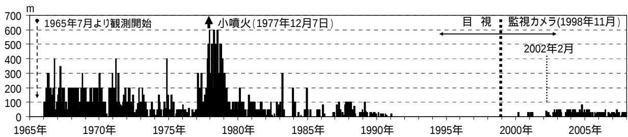
図2 吾妻山 月別最大噴気（噴煙）高（1965 年 7 月～2007 年 12 月）
