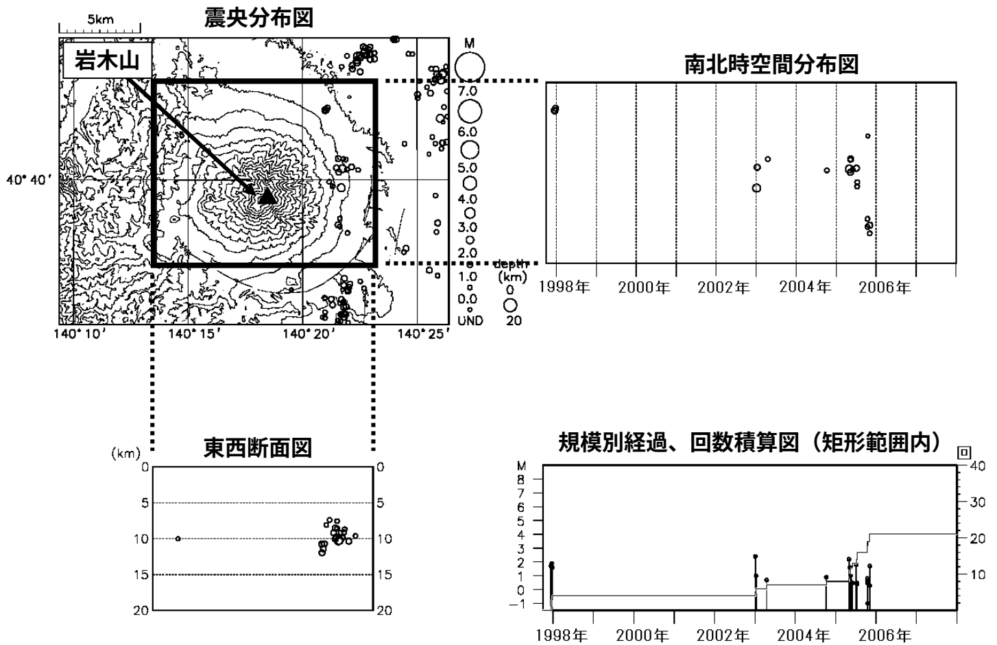
図 2※ 岩木山周辺の地震活動（1997 年 10 月～2007 年 12 月）
