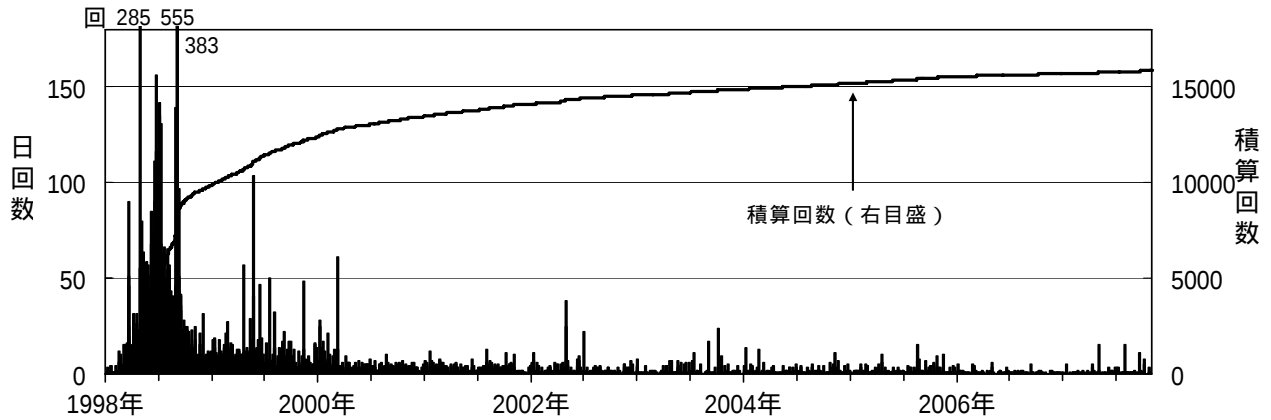
図 2 岩手山 日別地震回数（1998 年 1 月～2007 年 10 月）
