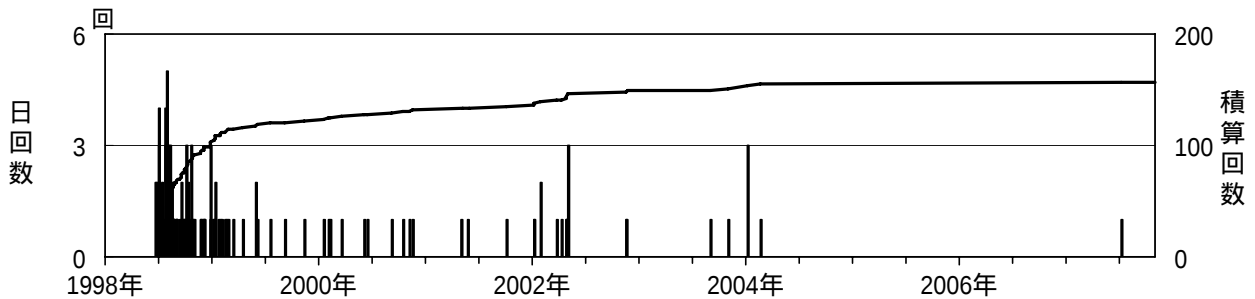
図 3 岩手山 日別微動回数（1998 年 1 月～2007 年 10 月）
