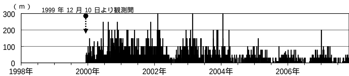
図 4 岩手山 日最大噴気の高さ（黒倉山）（1999 年 12 月 10 日～2007 年 10 月）
