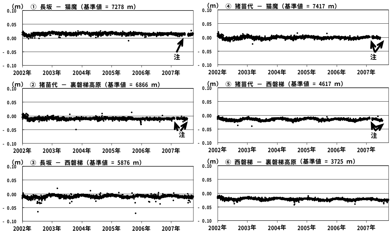
図 6 磐梯山 GPS 基線長変化図（2002 年 1 月～2007 年 9 月）
