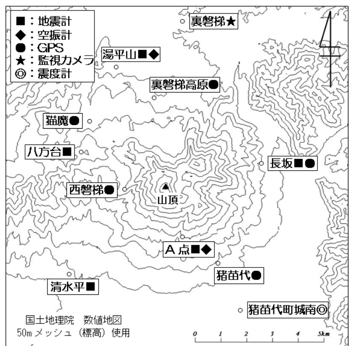
图1 磬梯山 观测点配置图
