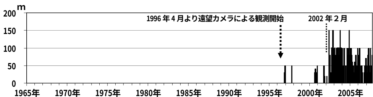
図 4 磐梯山 月最大噴気高（1996 年 4 月～2007 年 9 月）
