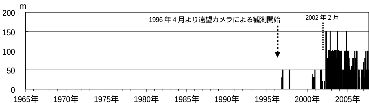
図 4 磐梯山 月最大噴気高（1996 年 4 月～2007 年 5 月）
