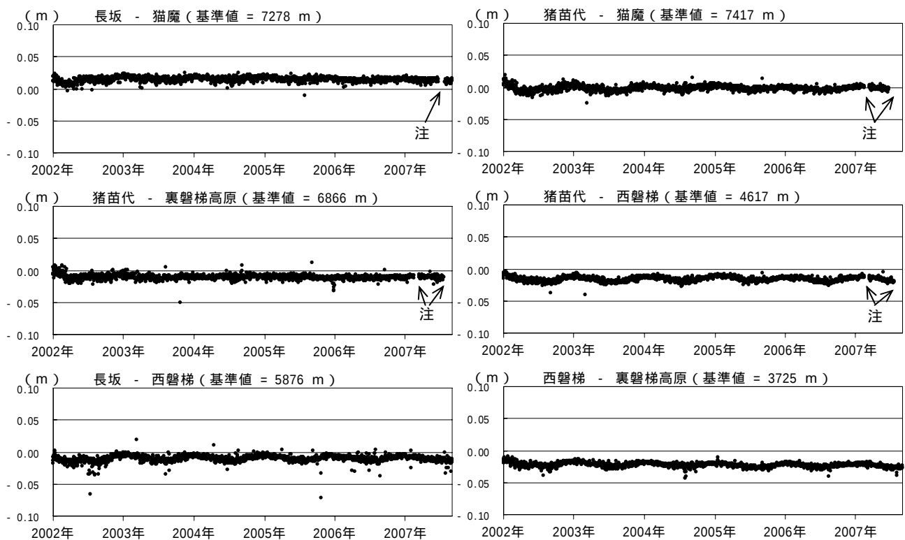
図 6 磐梯山 GPS 基線長変化図（2002 年 1 月～2007 年 8 月）
