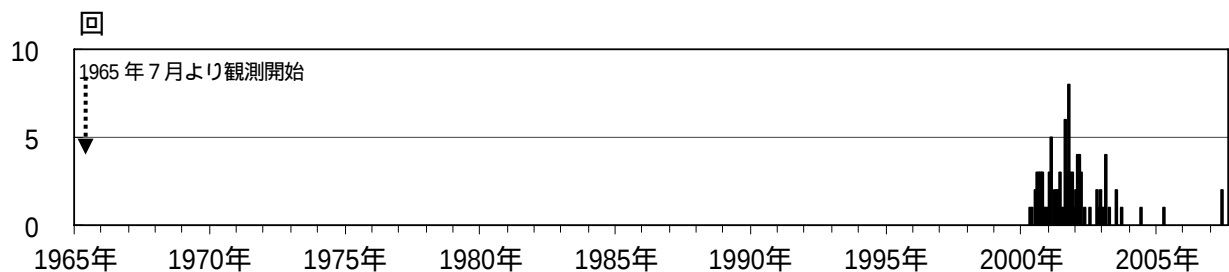
図 3 磐梯山 月別微動回数(1965 年 7 月～2007 年 8 月)
