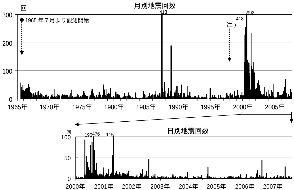
図 2 磐梯山 月別地震回数（1965 年 7 月～2007 年 8 月）
