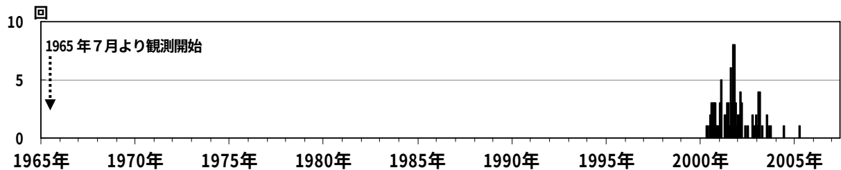
図 3 磐梯山 月別微動回数(1965 年 7 月～2007 年 5 月)
