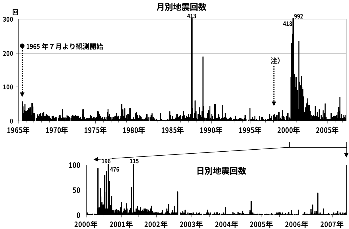
図 2 磐梯山 月別地震回数(1965 年 7 月～2007 年 5 月)
