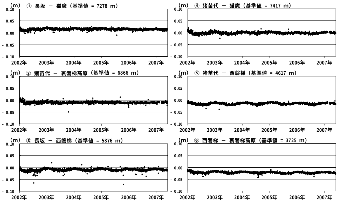
図 6 磐梯山 GPS 基線長変化図（2002 年 1 月～2007 年 5 月） ①～⑥は図 5 の GPS 基線①～⑥に対応しています。
