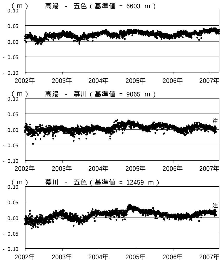
図 5 吾妻山 GPS 基線長変化図 (2002 年 1 月 ~ 2007 年 3 月)
