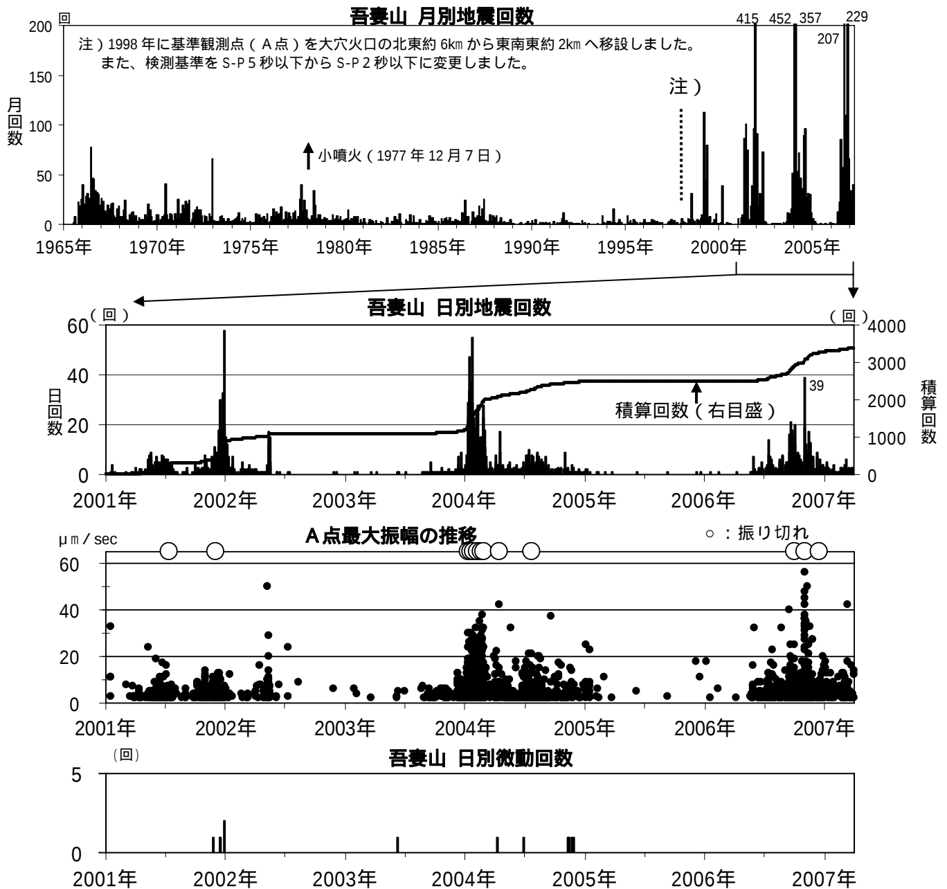
図3 吾妻山の地震回数および微動回数
