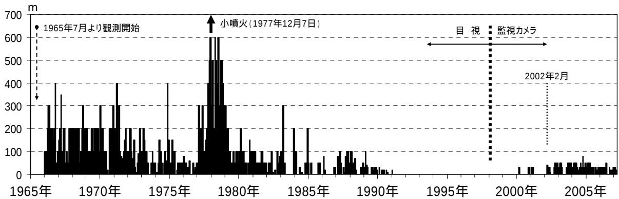
図2 吾妻山 月別最大噴気(噴煙)高(1965年7月～2007年3月)
