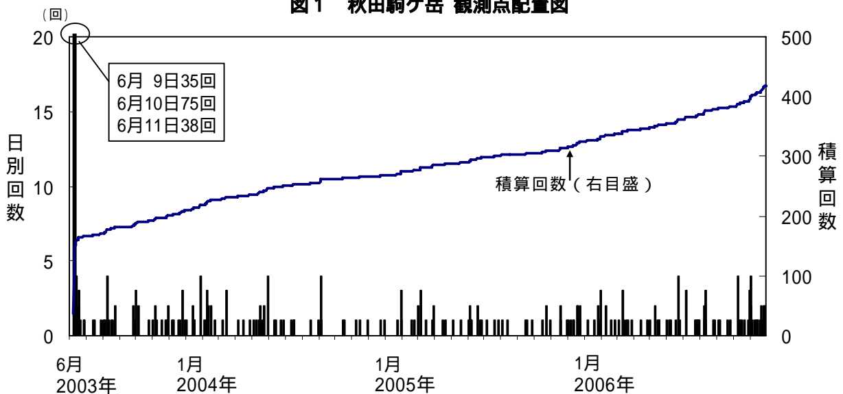
図2 秋田駒ヶ岳 日別地震回数(2003年6月9日~2006年11月)
