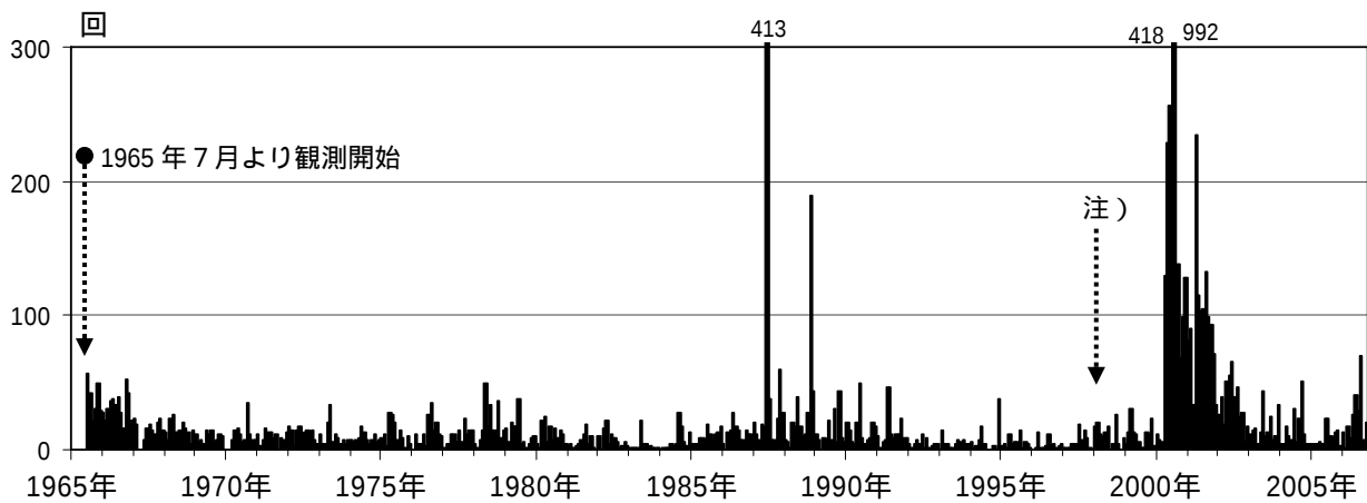
図2 磐梯山 月別地震回数(1965年7月～2006年10月)
