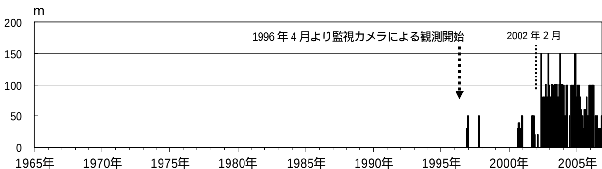
図4 磐梯山 月最大噴気高 (1996年4月～2006年10月)
