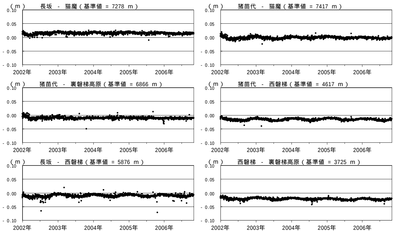
図6 磐梯山 GPS 基線長変化図 (2002年1月～2006年10月)
