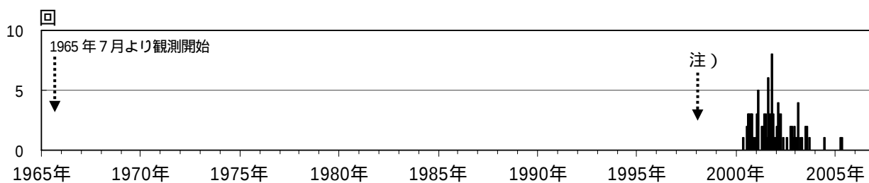
図3 磐梯山 月別微動回数(1965年7月～2006年10月)
