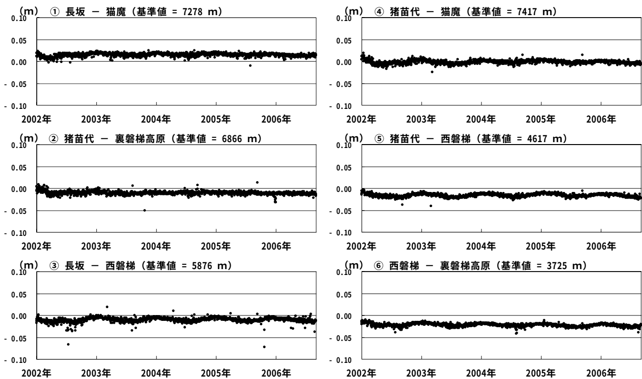
図6 磐梯山 GPS 基線長変化図（2002年1月～2006年9月）
