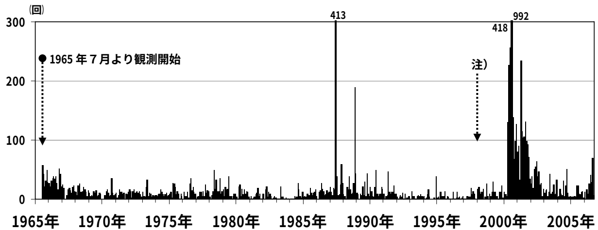
図2 磐梯山 月別地震回数(1965年7月～2006年9月)
