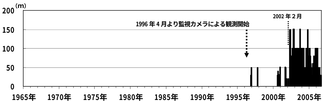
図4 磐梯山 月最大噴気高 (1996年4月～2006年9月)
