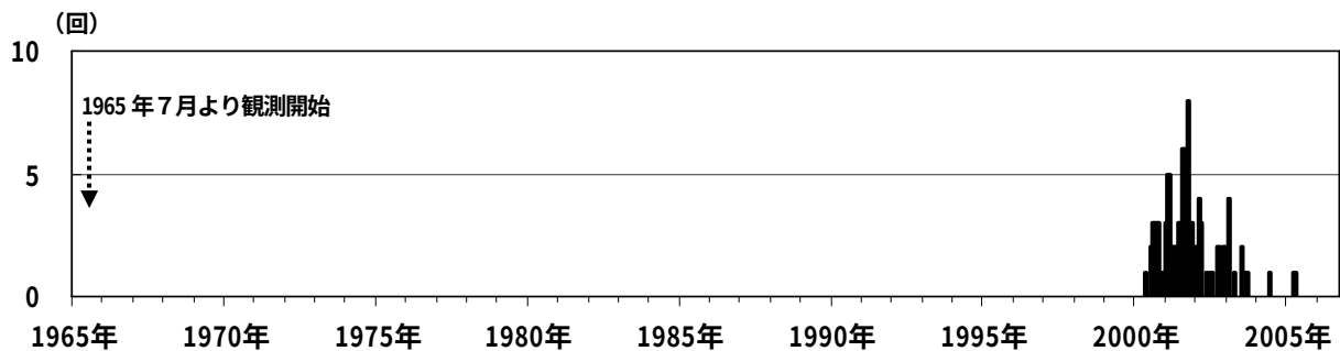
図3 磐梯山 月別微動回数(1965年7月～2006年9月)
