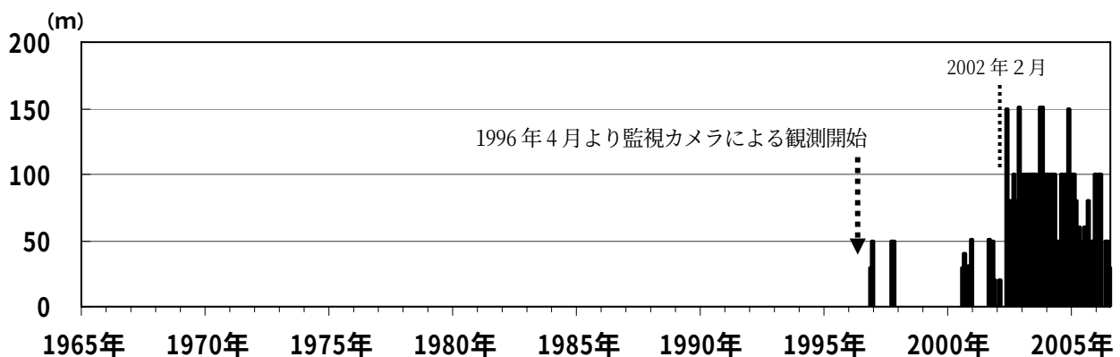
図4 磐梯山 月最大噴気高 (1996年4月～2006年7月)
