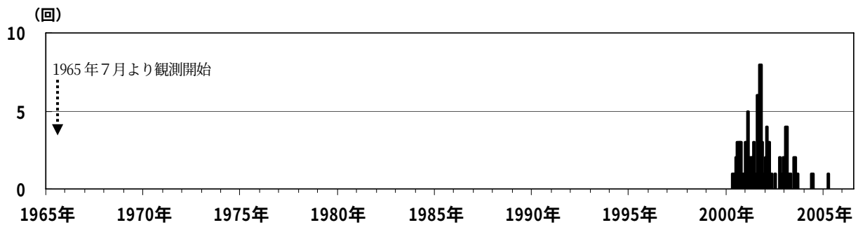
図3 磐梯山 月別微動回数(1965年7月～2006年7月)
