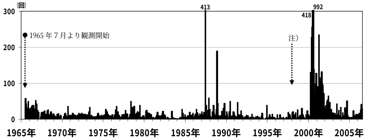
図2 磐梯山 月別地震回数(1965年7月～2006年7月)
