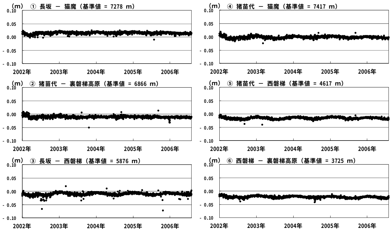
図6 磐梯山 GPS 基線長変化図（2002年1月～2006年7月）
