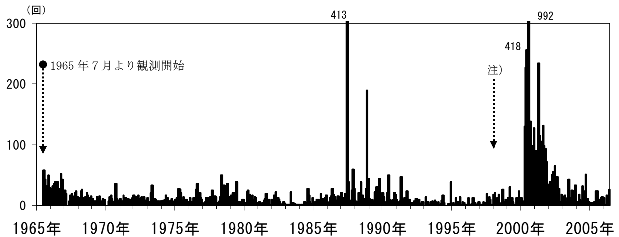
図 2 磐梯山 月別地震回数(1965 年 7 月～2006 年 5 月)
