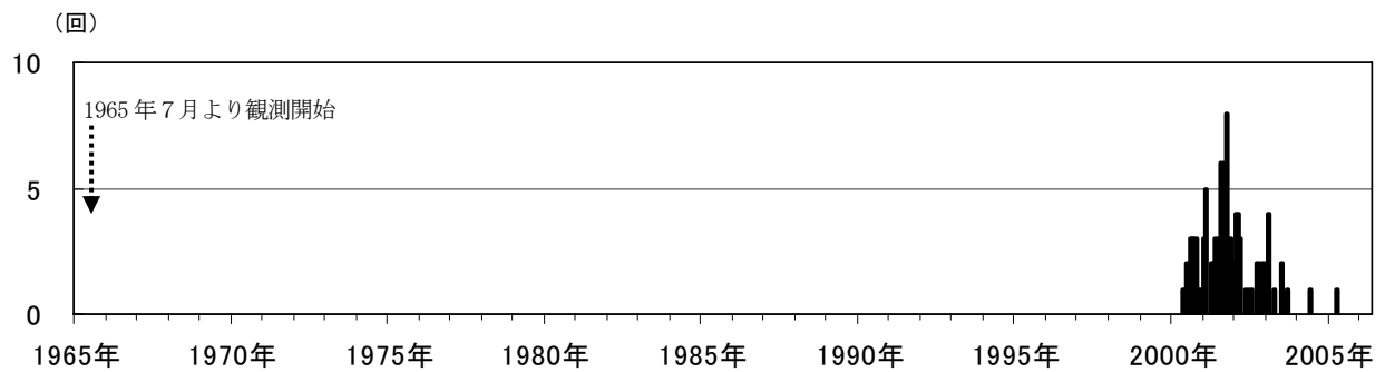
図 3 磐梯山 月別微動回数(1965 年 7 月～2006 年 5 月)
