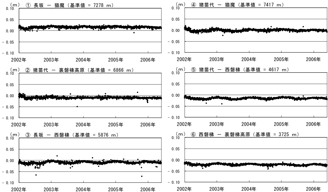
図6 磐梯山 GPS 基線長変化図（2002年1月～2006年5月）
