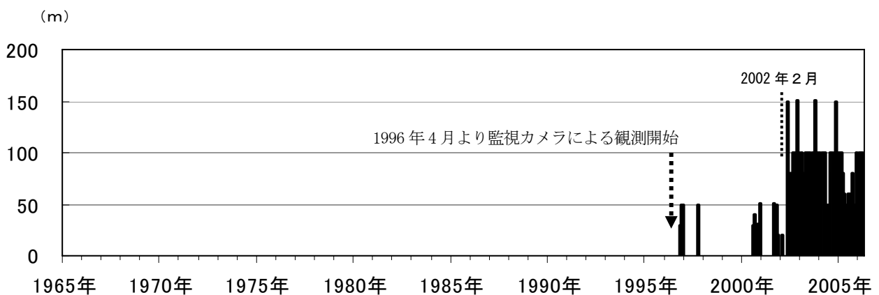
図 4 磐梯山 月最大噴気高 (1996 年 4 月～2006 年 4 月)
