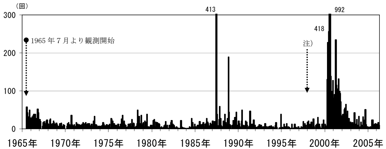
図 2 磐梯山 月別地震回数(1965 年 7 月～2006 年 4 月)
