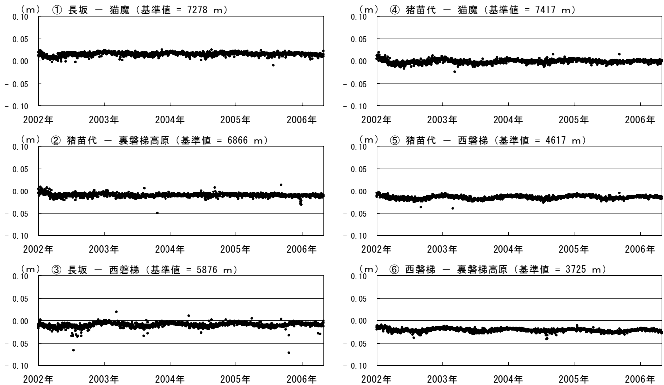
図6 磐梯山 GPS 基線長変化図（2002年1月～2006年4月）
