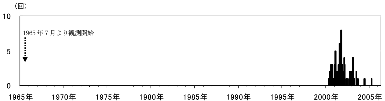
図 3 磐梯山 月別微動回数(1965 年 7 月～2006 年 4 月)
