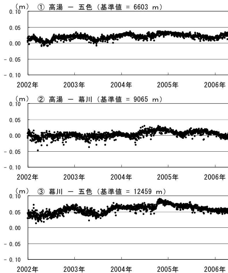
図5 吾妻山 GPS 基線長変化図 (2002年1月～2006年4月)
