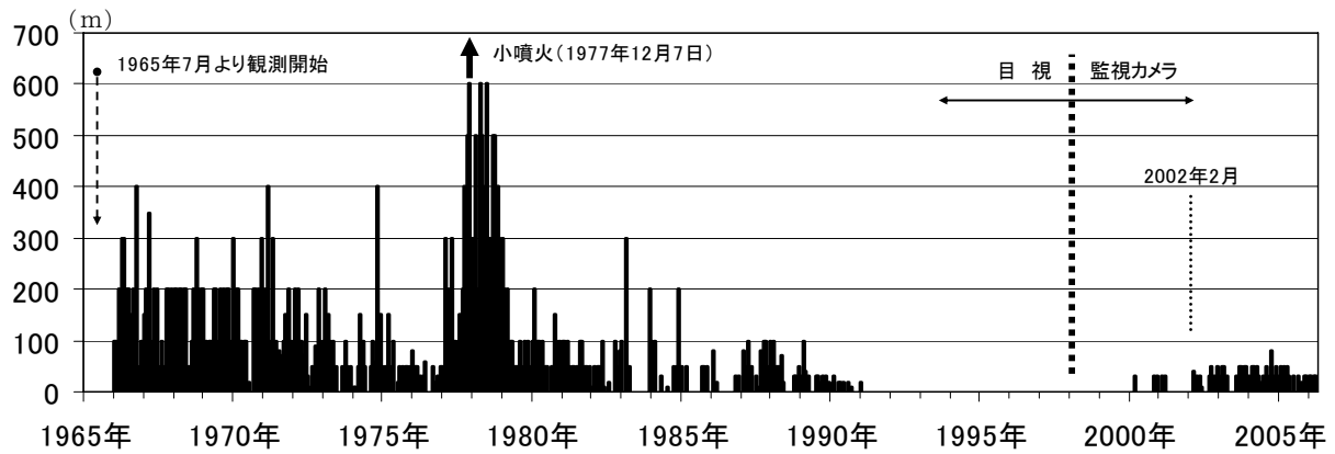
図2 吾妻山 月別最大噴気(噴煙)高(1965年7月～2006年4月)
