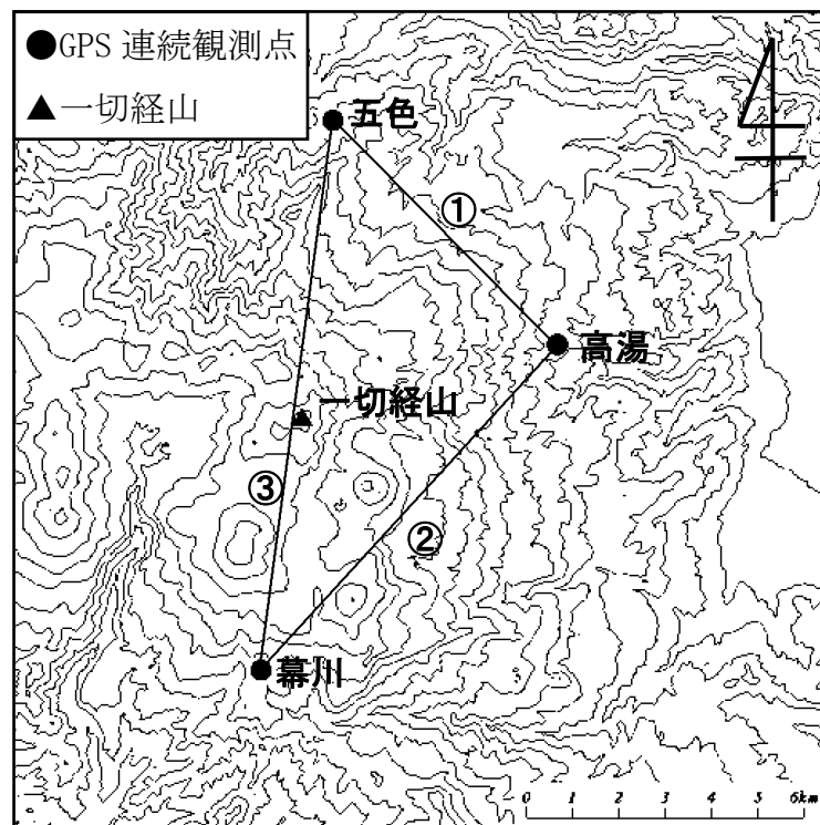
図4** 吾妻山 GPS 観測点配置図
