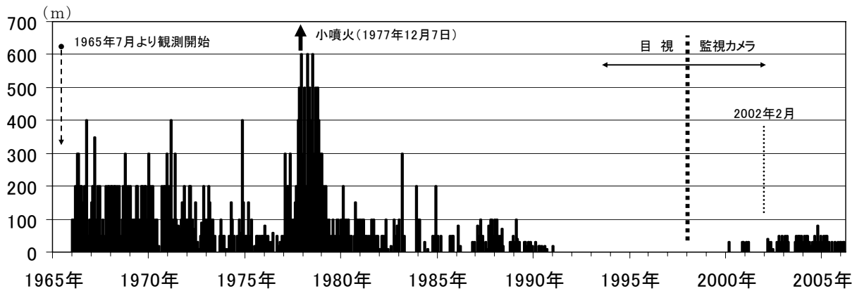
図2 吾妻山 月別最大噴気(噴煙)高(1965年7月～2006年3月)
