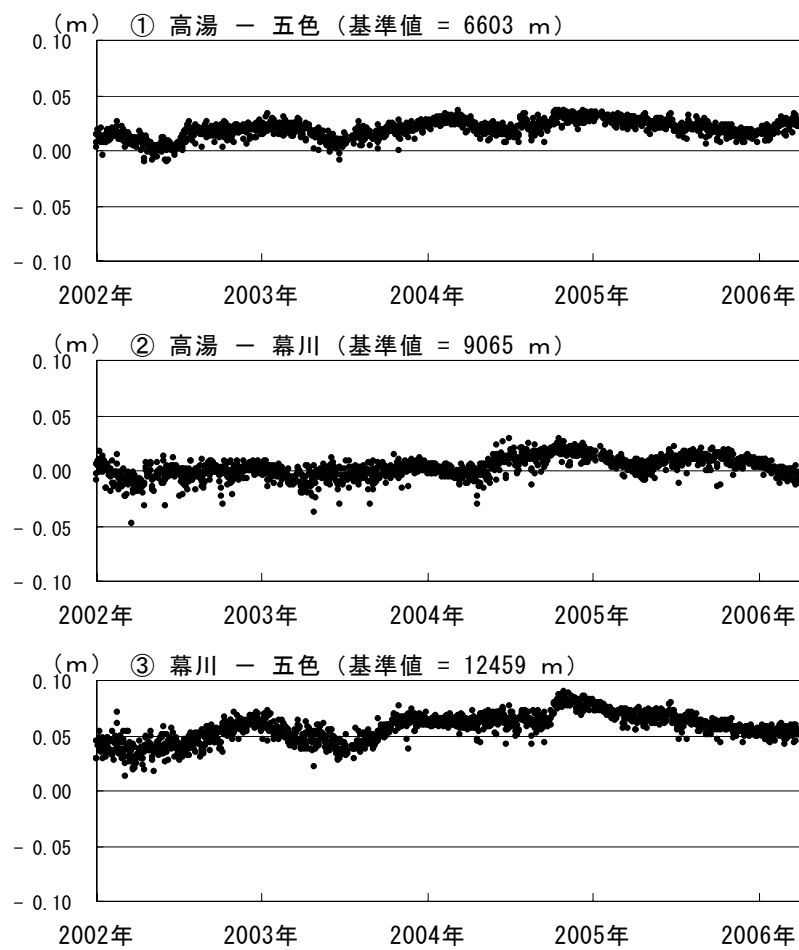
図5 吾妻山 GPS 基線長変化図 (2002年1月～2006年3月)
