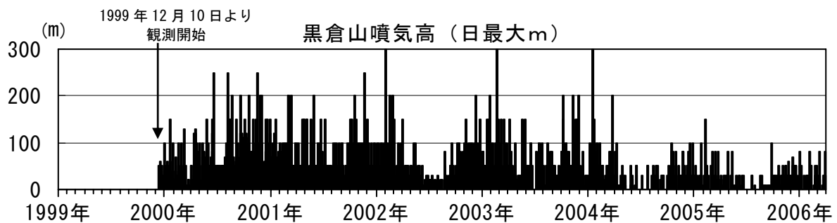
図2 岩手山 日最大噴気の高さ（黒倉山）
