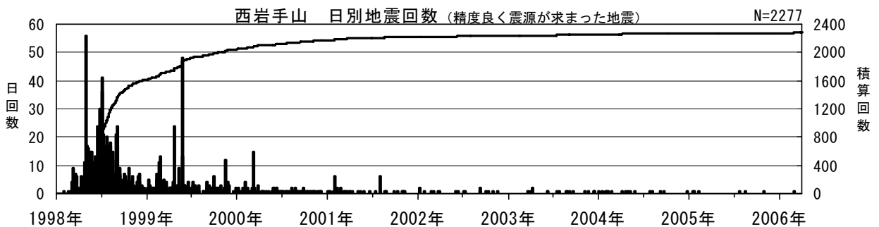
図4※ 東岩手山、西岩手山 日別地震回数 (1998年1月～2006年3月)
