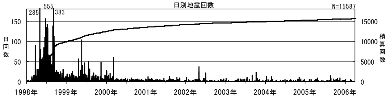
図3※ 岩手山 日別地震回数 (1998年1月～2006年3月)
