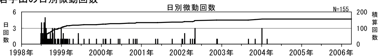
図5※ 岩手山 日別微動回数 (1998年1月～2006年3月)
