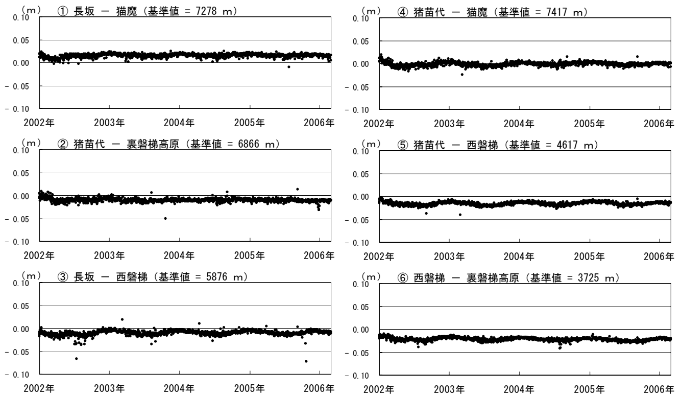
図6 GPS基線長変化図（2002年1月～2006年2月）
