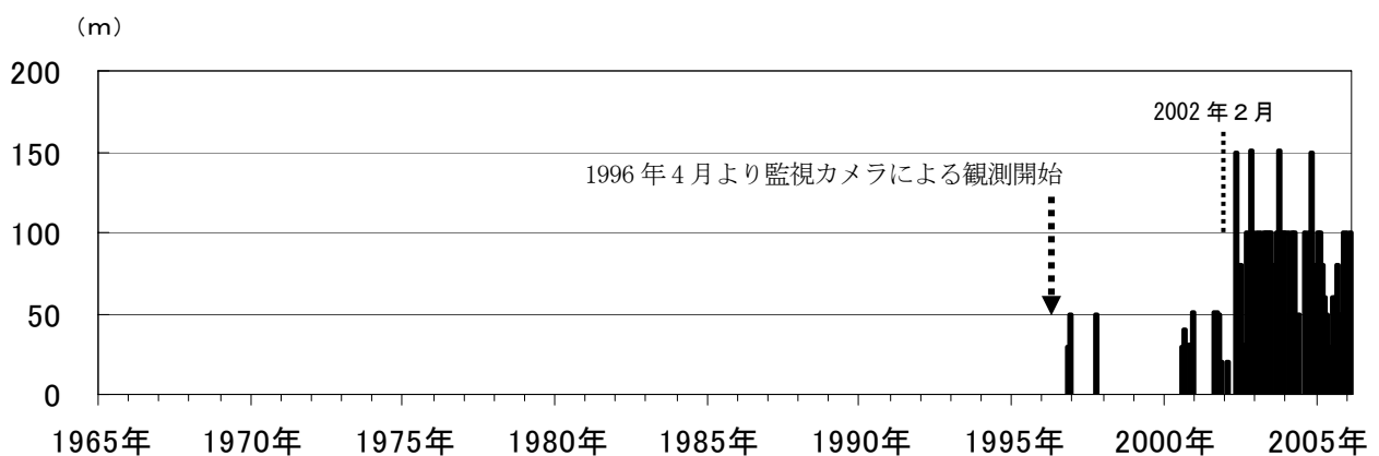
図4 磐梯山月最大噴気高 (1996年4月～2006年2月)
