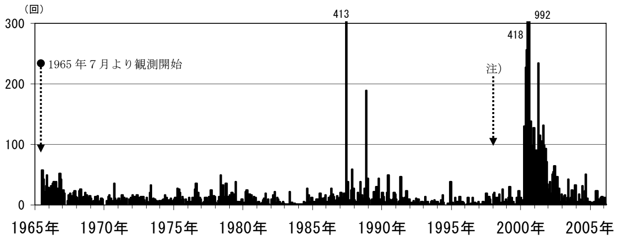
図2 磐梯山月別地震回数(1965年7月～2006年2月)
