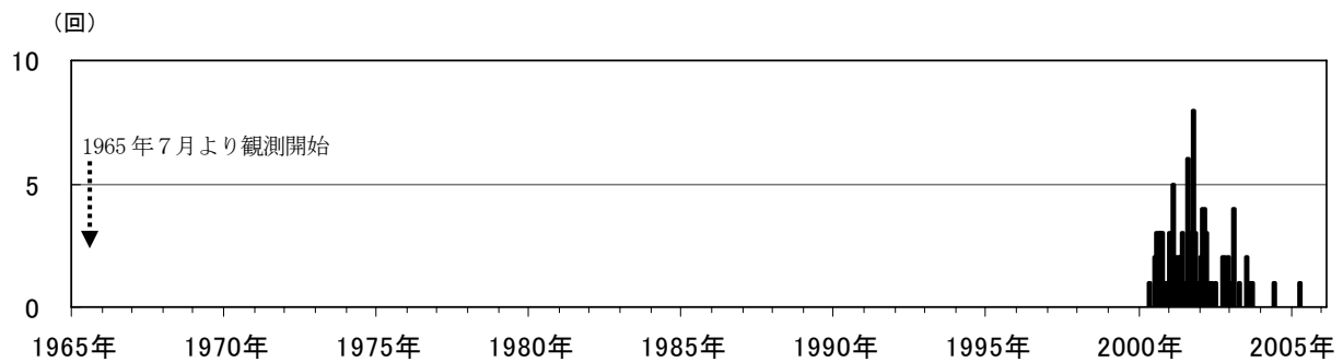
図3 磐梯山月別微動回数(1965年7月～2006年2月)
