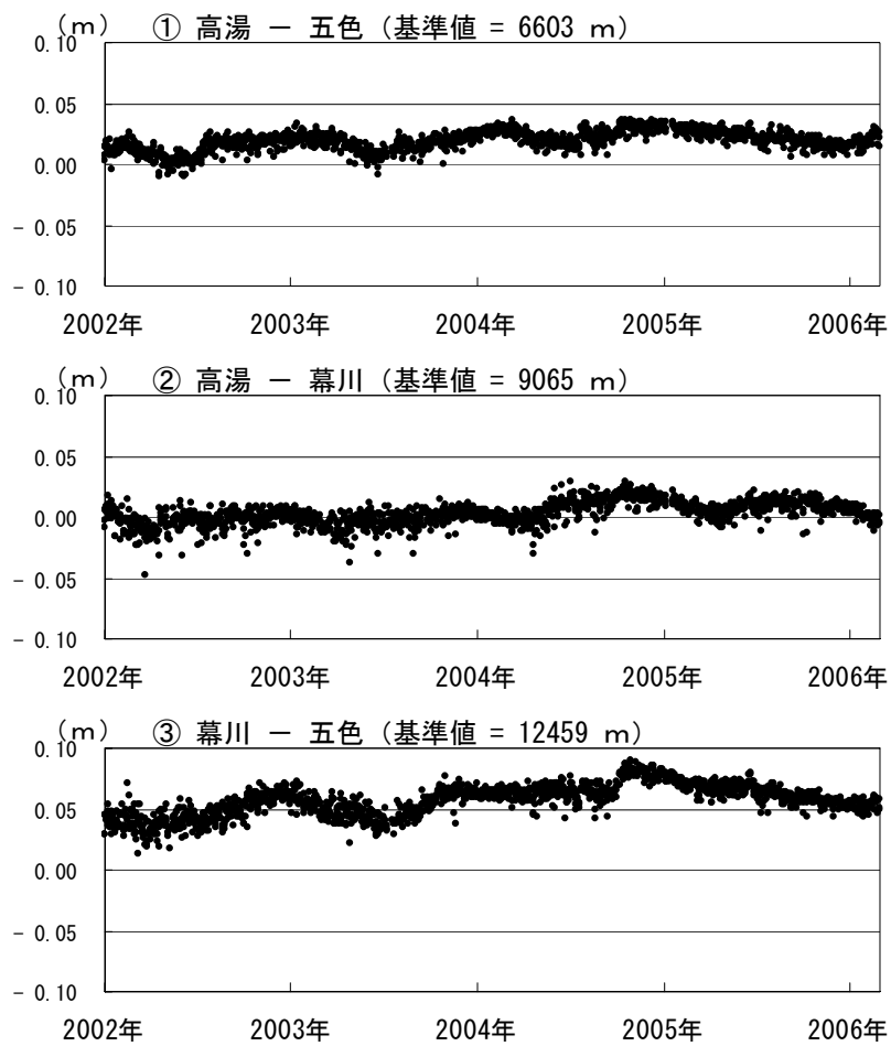
図5 GPS 基線長変化図 (2002年1月～2006年2月)
