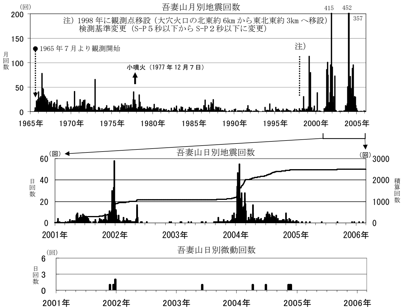
図3 吾妻山の地震回数および微動回数
