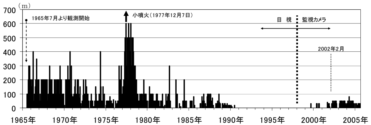
図2 吾妻山月別最大噴気(噴煙)高(1965年7月～2006年2月) 1998年より監視カメラによる観測(1997年以前は福島地方気象台から目視観測) 2002年2月以前は定時(09時, 15時)及び随時観測による高さ。 2002年2月以後は全ての時間を収録データから観測した高さ。
