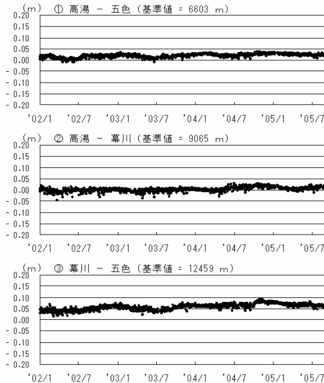
GPS 基線長変化図 (2002.1 ~ 2005.8)
