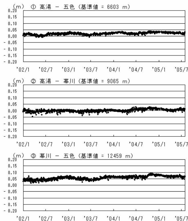
GPS 基線長変化図 (2002.1 ~ 2005.7)
