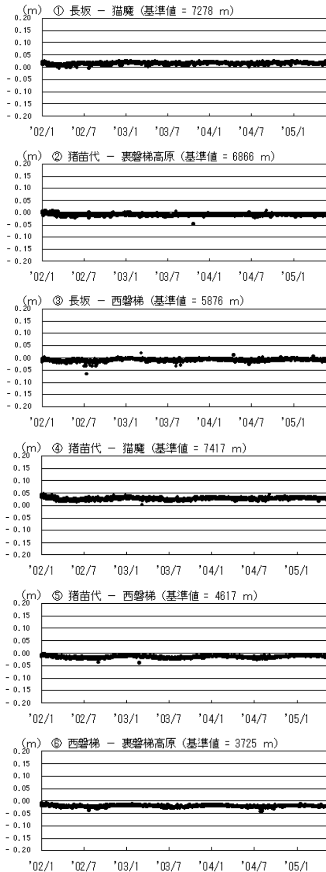
G P S 基線長変化図 (2002. 1～2005. 5)
