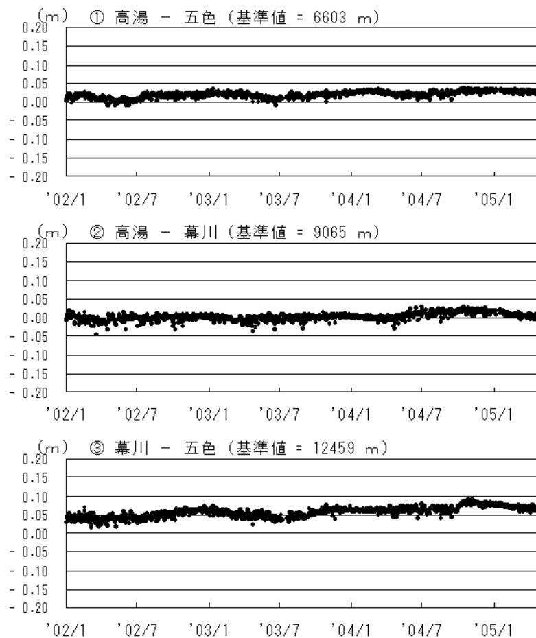
G P S 基線長変化図（2002. 1～2005. 4）
