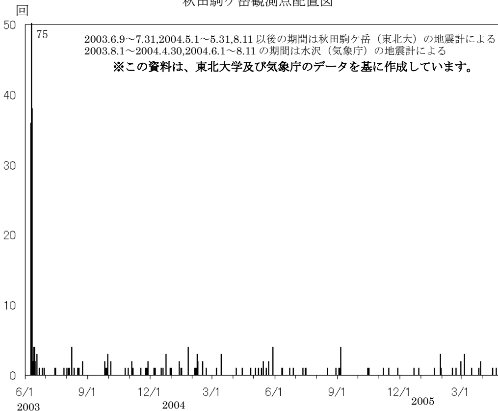
秋田駒ヶ岳日別地震回数 (2003. 6. 9~2005. 4. 30)
