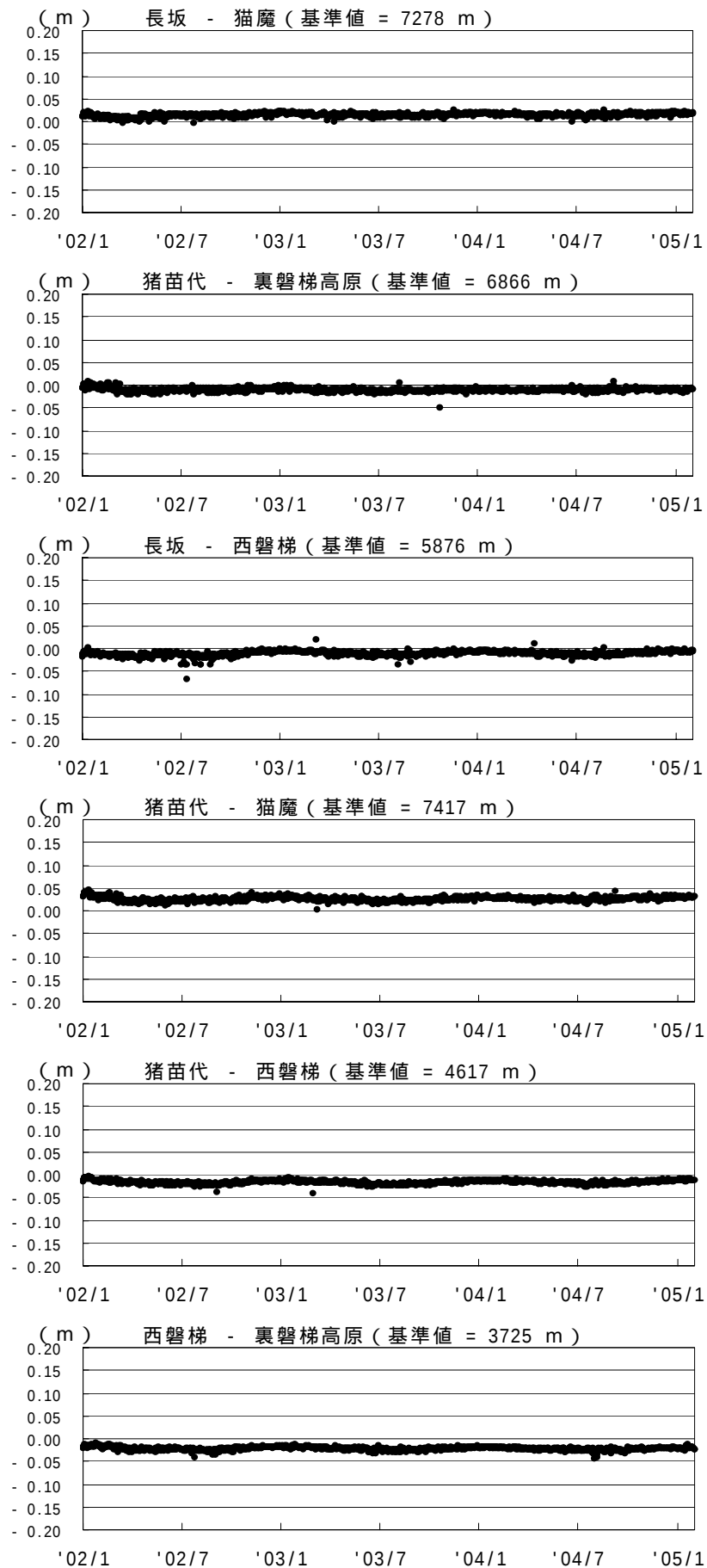
G P S 基線長变化図 (2002.1 ~ 2005.1)
