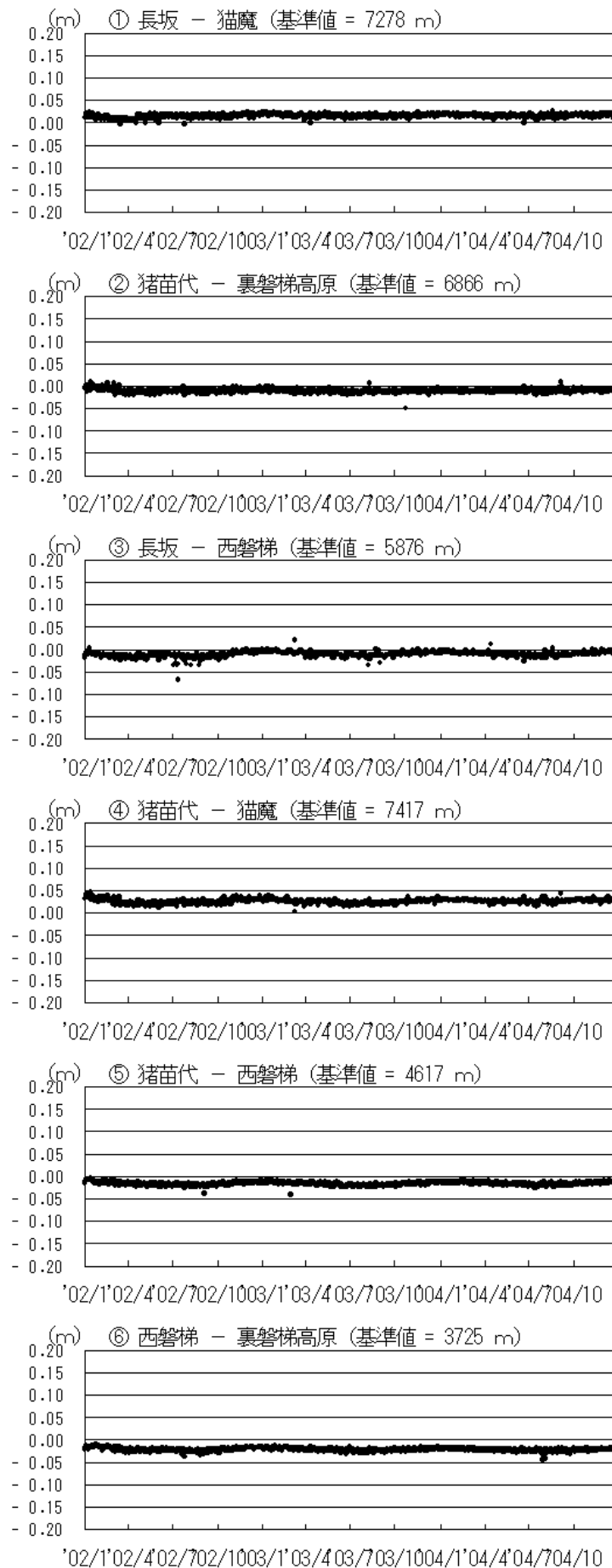
G P S 基線長変化図 (2002. 1 ~ 2004. 12)
