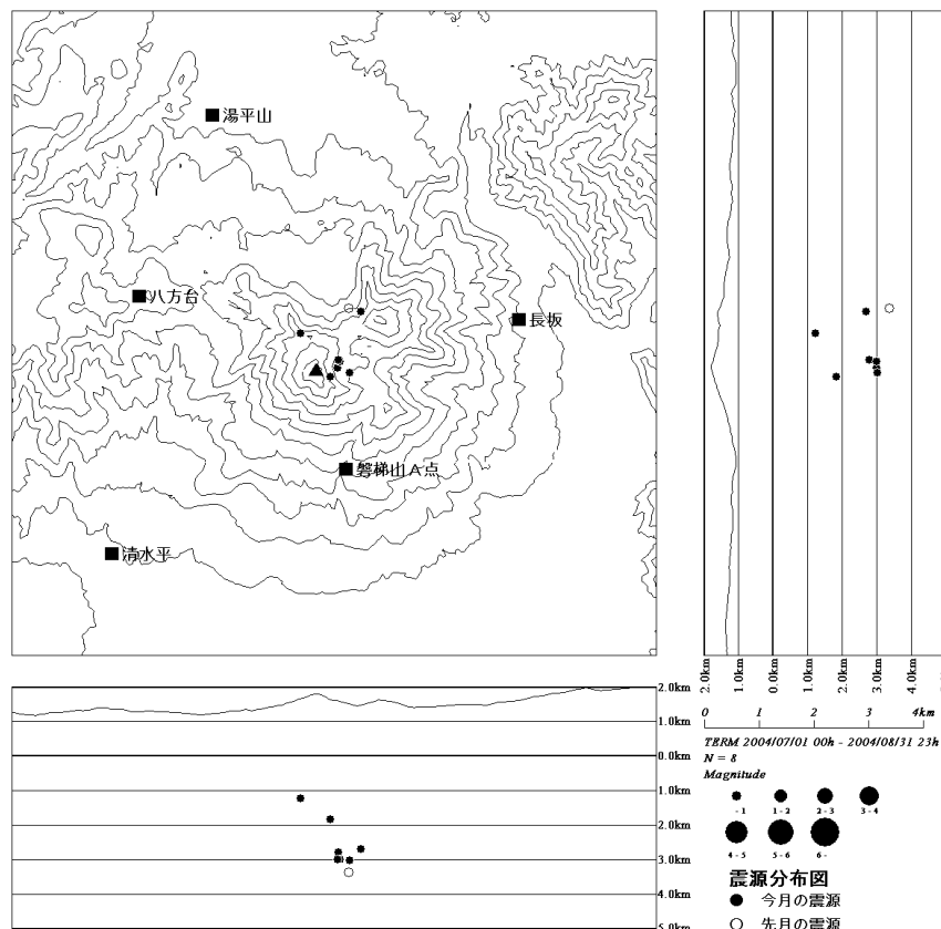
磐梯山震源分布図(2004. 7. 1～2004. 8. 31)
