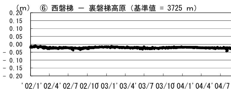
GPS 基線長変化図（2002.1～2004.8）
