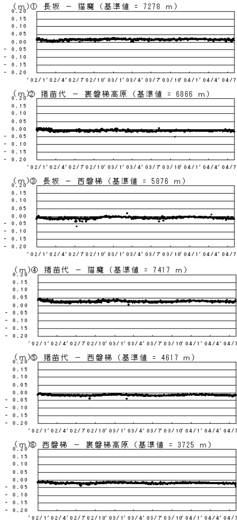
GPS 基線長変化図（2002.1～2004.7）
