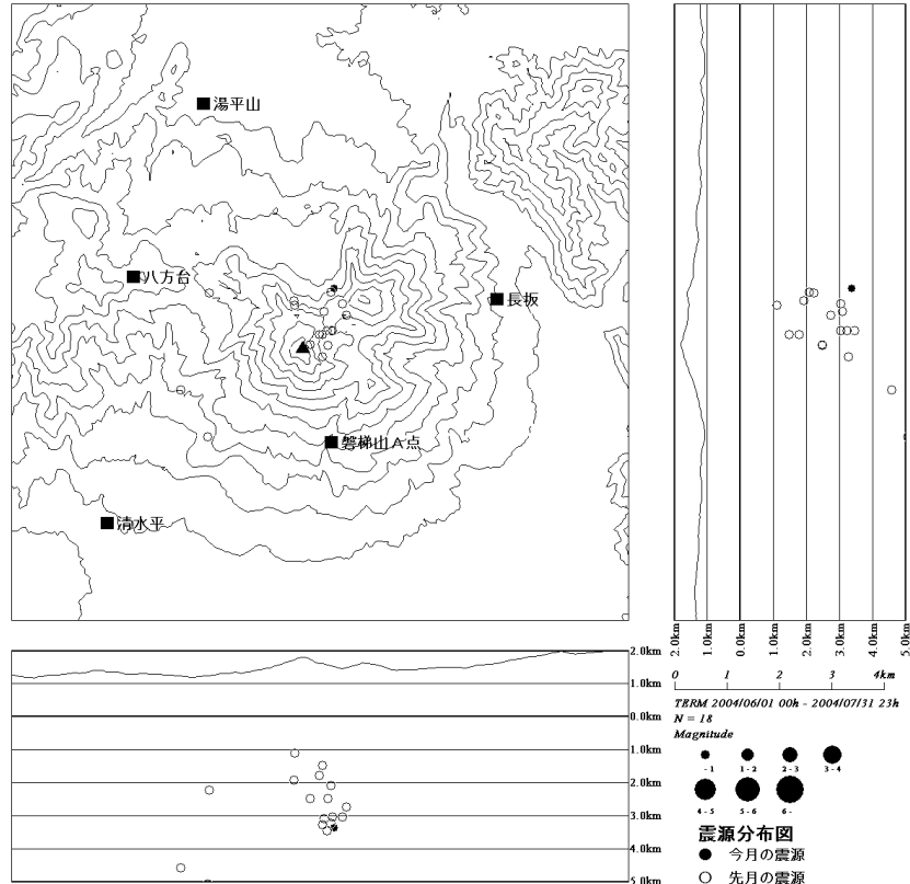
磐梯山震源分布図(2004. 6. 1～2004. 7. 31)
