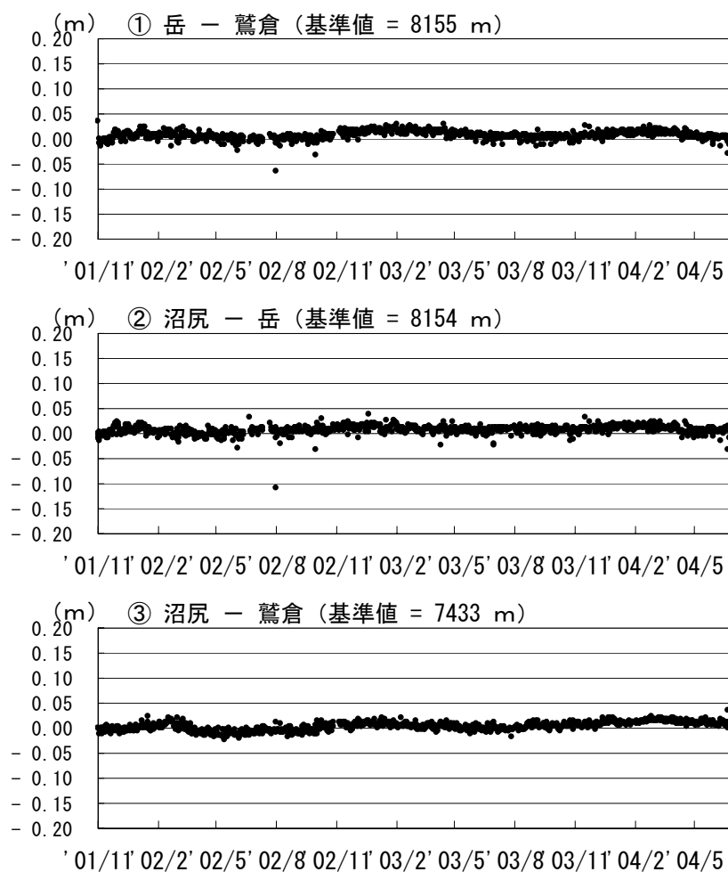
GPS 基線長変化図 (2002. 1~2004. 6)
