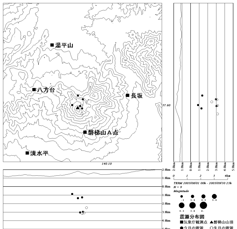
磐梯山震源分布図(2003.8.1～9.30)
