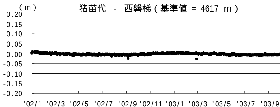
GPS 基線長変化図 (2002.1 ~ 2003.9)
