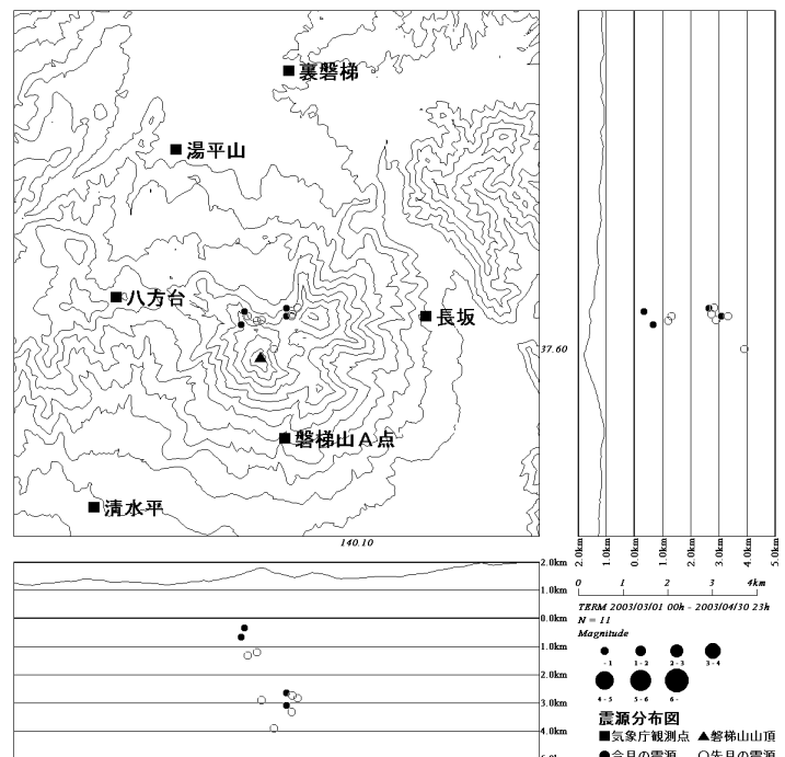
磐梯山震源分布図(2003. 03. 01～04. 30)
