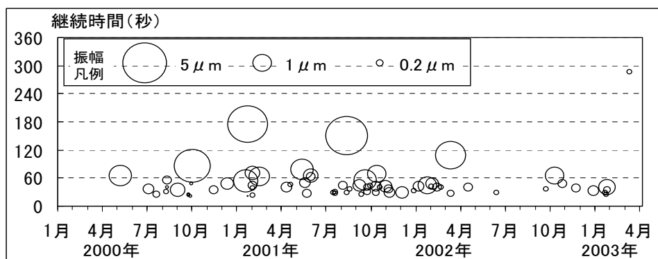
磐梯山微動の最大振幅（U/D）と継続時間（2000 年 1 月～2003 年 4 月）
