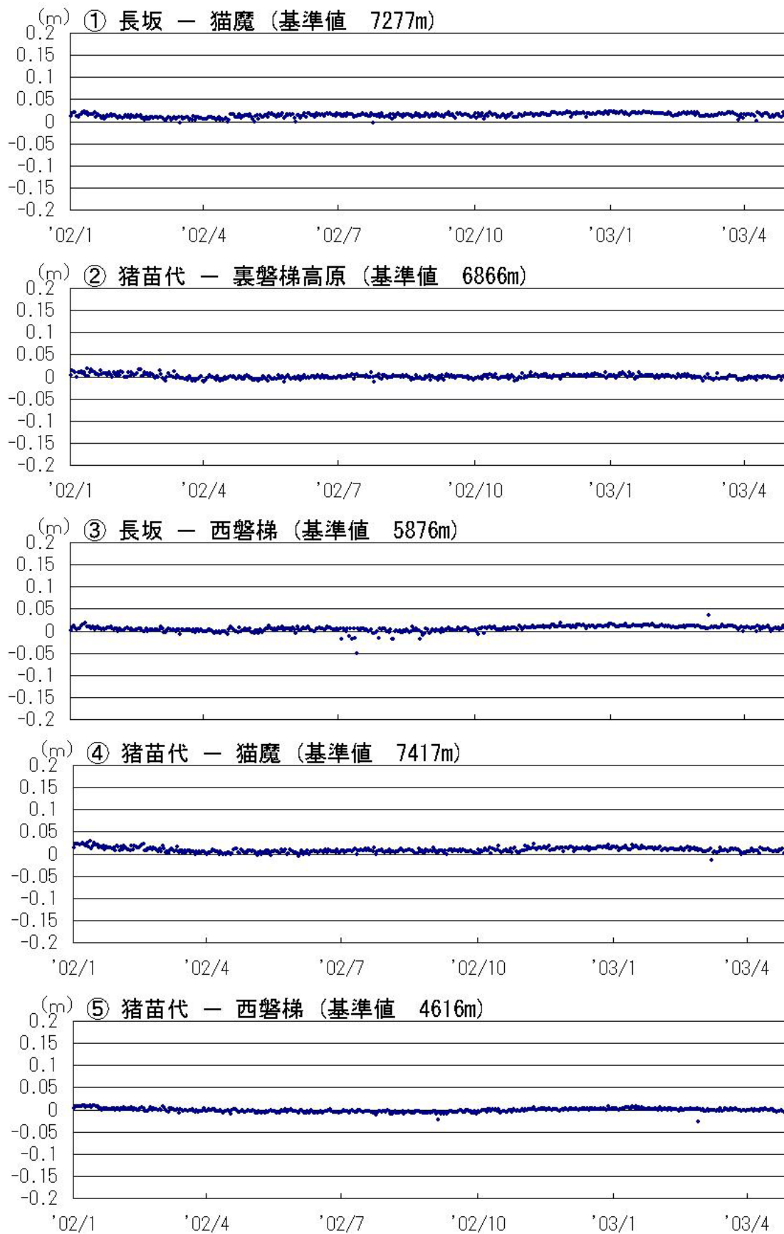
GPS 基線長変化図 (2002. 01～2003. 04)
