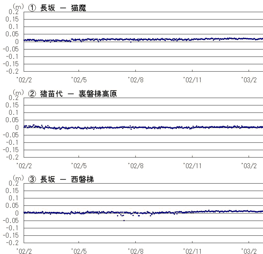
GPS 基線長変化図 (2002.02 ~ 2003.02)
