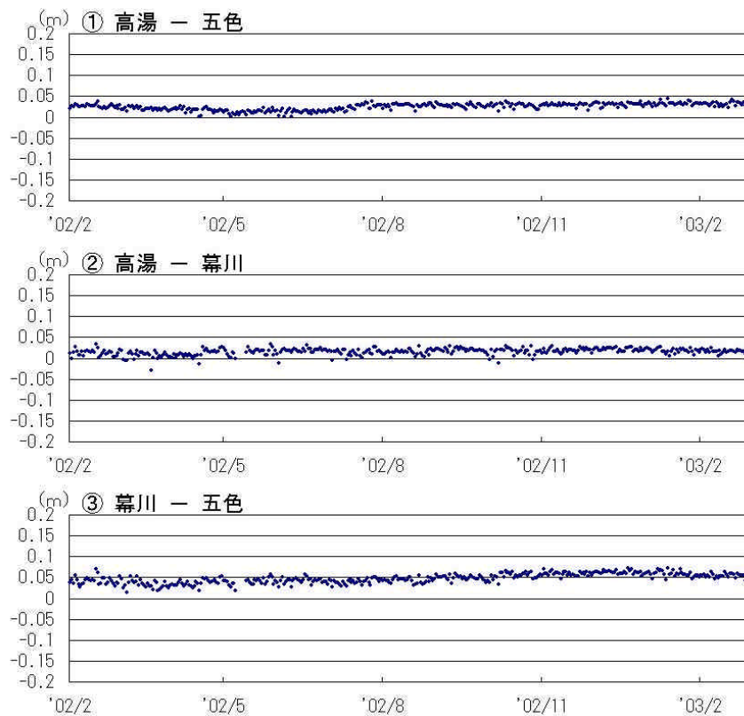
GPS 基線長変化図 (2002.02 ~ 2003.02)
