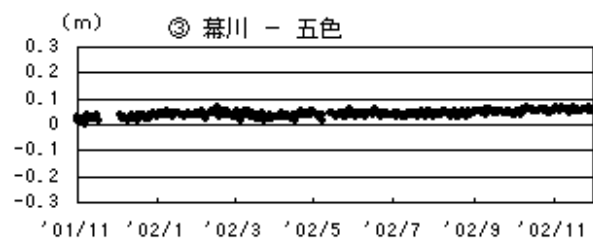
GPS 基線長変化図 (2001.11 ~ 2002.11)
