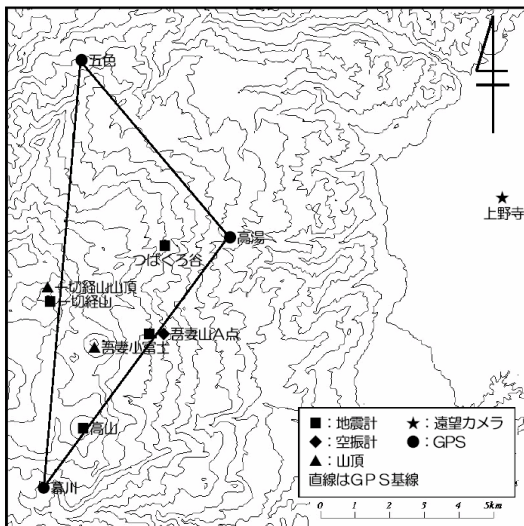
吾妻山火山観測点配置図
