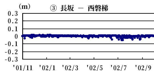
GPS 基線長変化図 (2001.11～2002.09)
