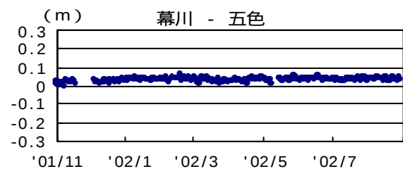
GPS 基線長変化図 (2001.11 ~ 2002.08)
