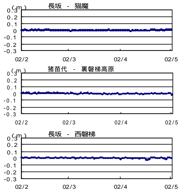
GPS 基線長変化図 (2002.2 ~ 2002.5)
