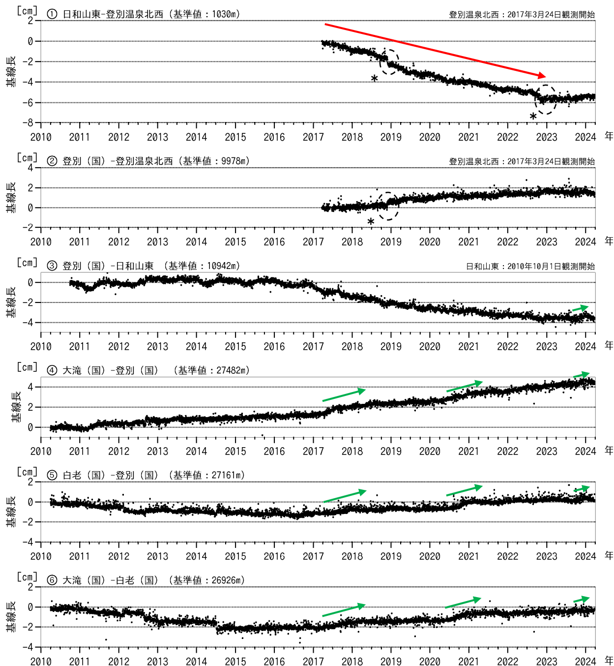
図3 倶多楽 GNSS連続観測による基線長変化 (2010年4月～2024年3月)
