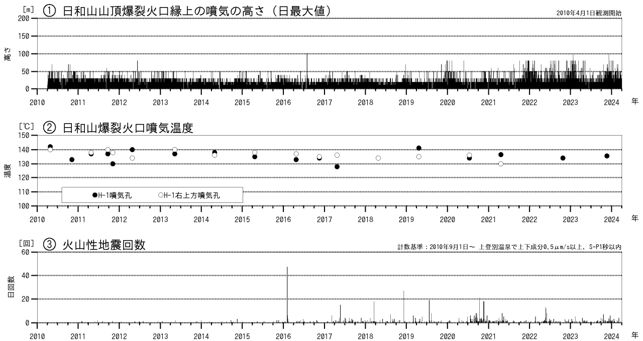
図2 倶多楽 火山活動経過図 (2010年1月～2024年3月)
