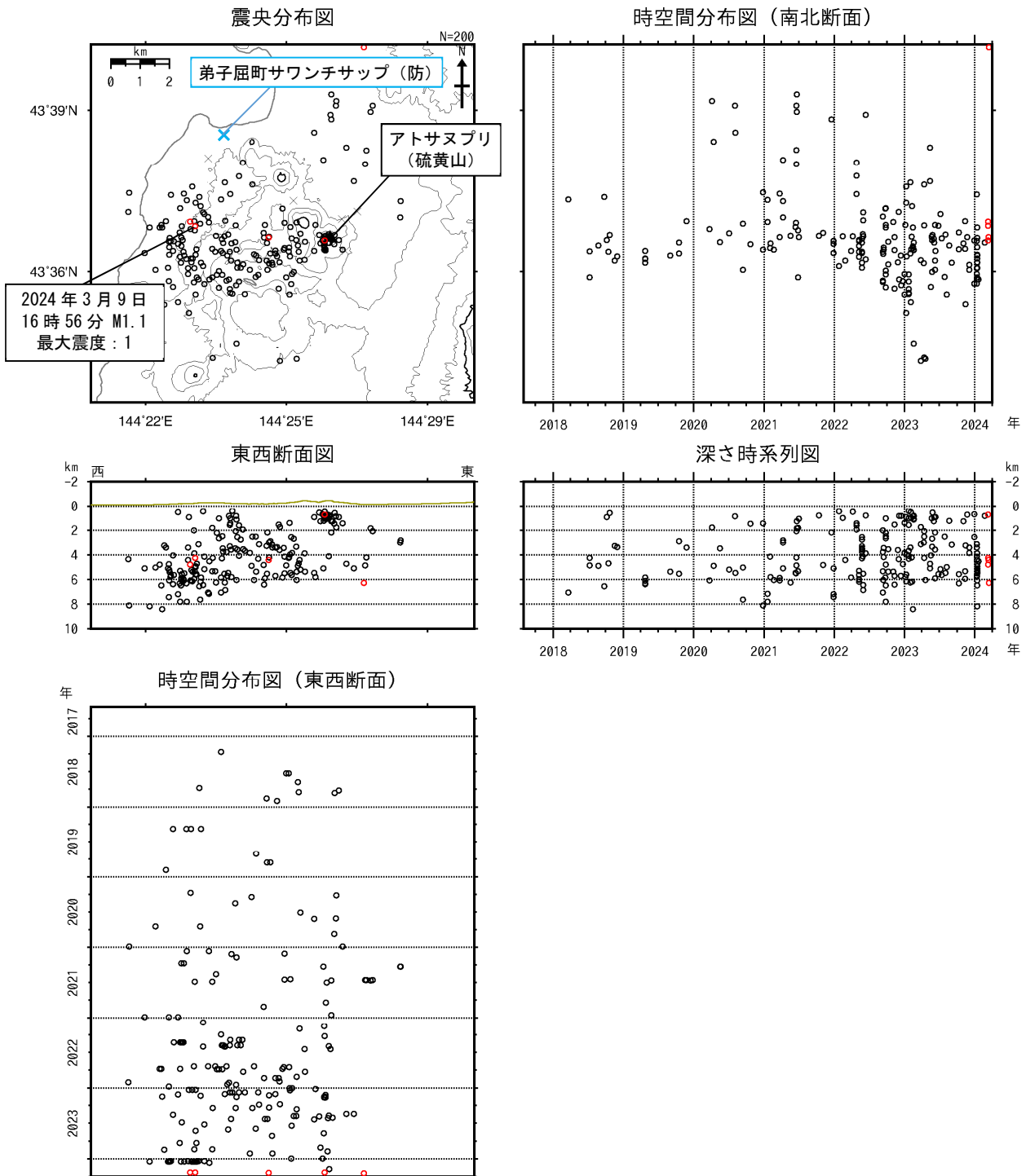
図3 アトサヌプリ 火山性地震の震源分布 (2017年8月~2024年3月)
