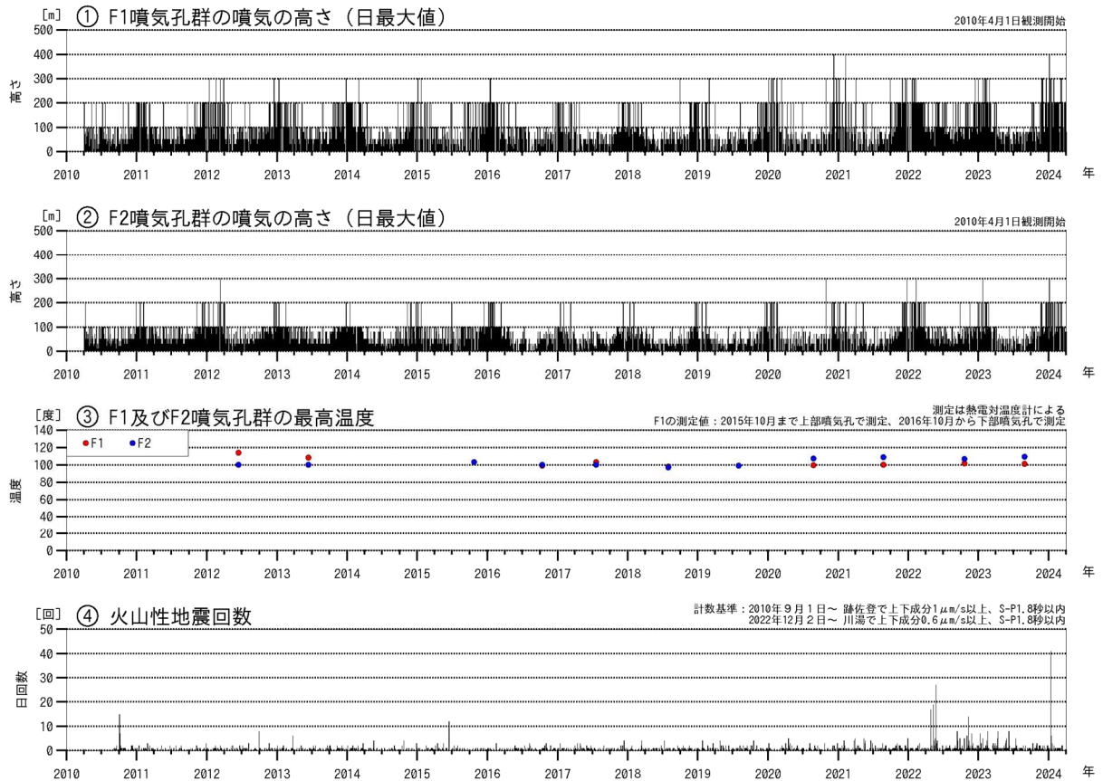
図1 アトサヌプリ 火山活動経過図（2010年4月～2024年3月）
