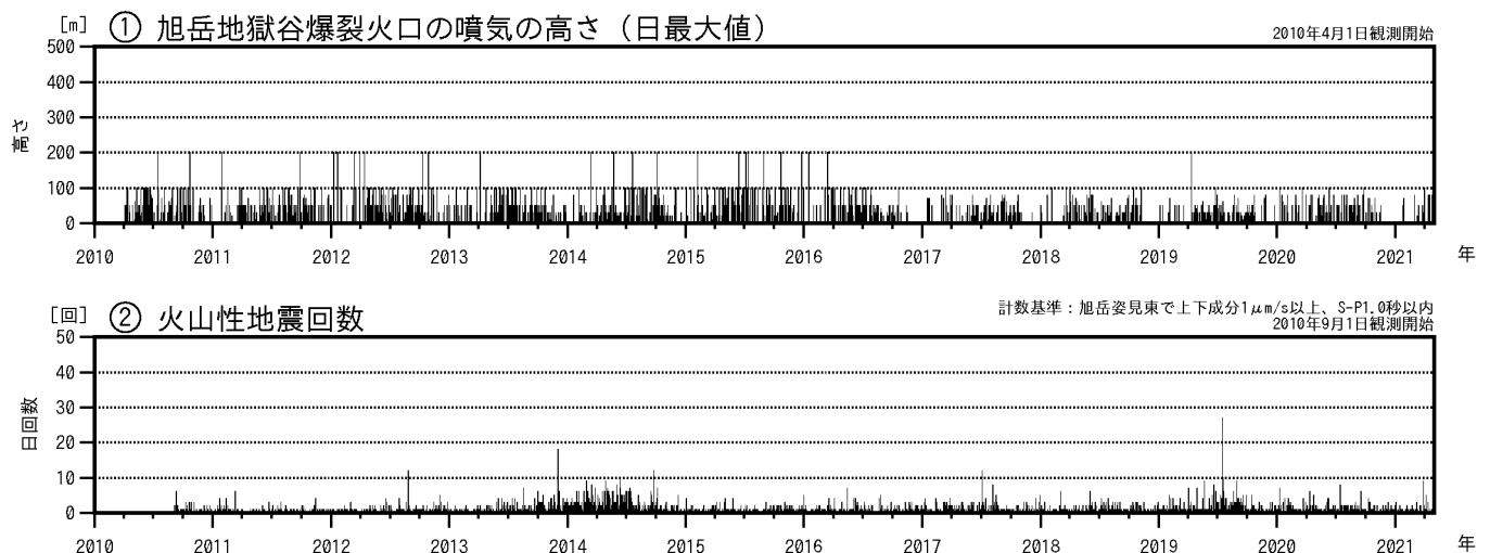
図1 大雪山 火山活動経過図（2010年4月～2021年4月）
