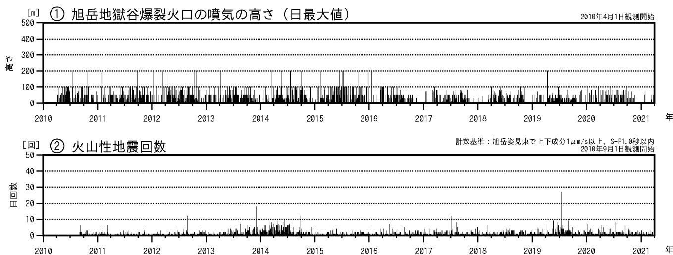
図1 大雪山 火山活動経過図（2010年4月～2021年3月）
