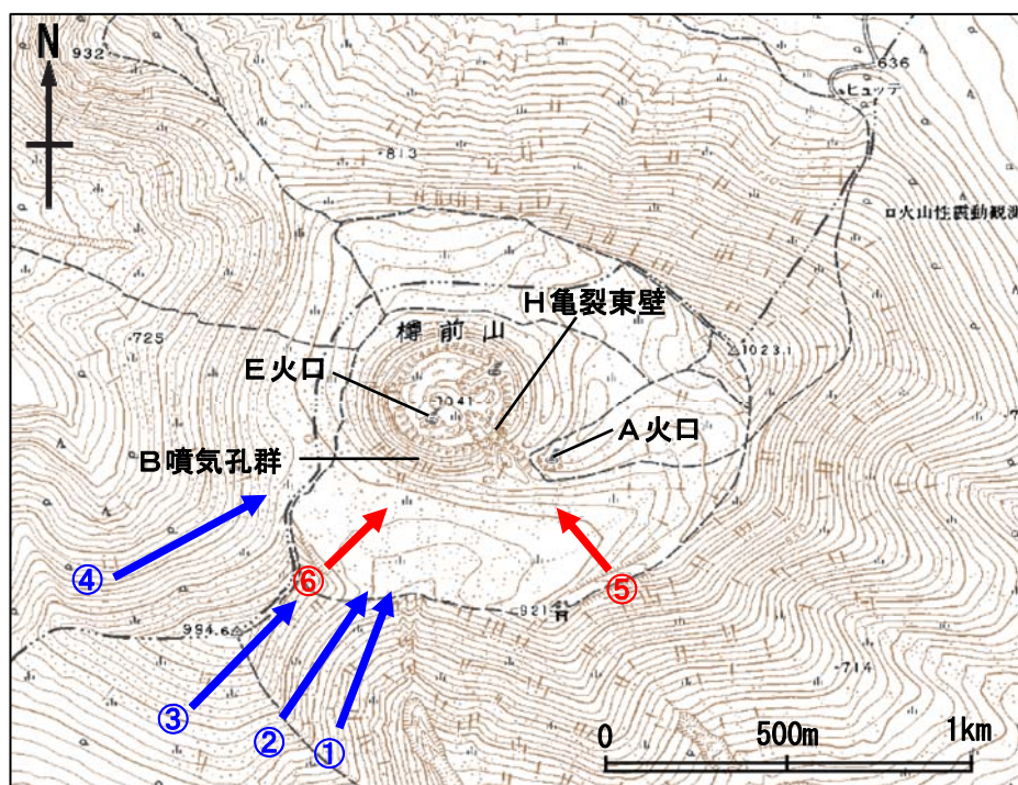
図 3 樽前山 写真及び赤外熱映像の撮影方向 (矢印) ・青矢印は上空からの撮影、赤矢印は地上からの撮影を示します
