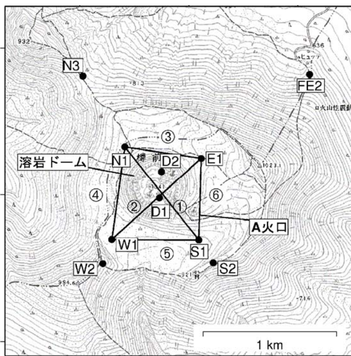
図11 樽前山 GNSS繰り返し観測による山頂溶岩ドーム付近の基線長変化(1999年7月～2017年5月)及び観測点配置図
