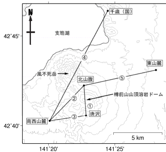
図10 樽前山 GNSS連続観測による基線長変化 (2005年1月~2017年12月) 及び観測点配置図
