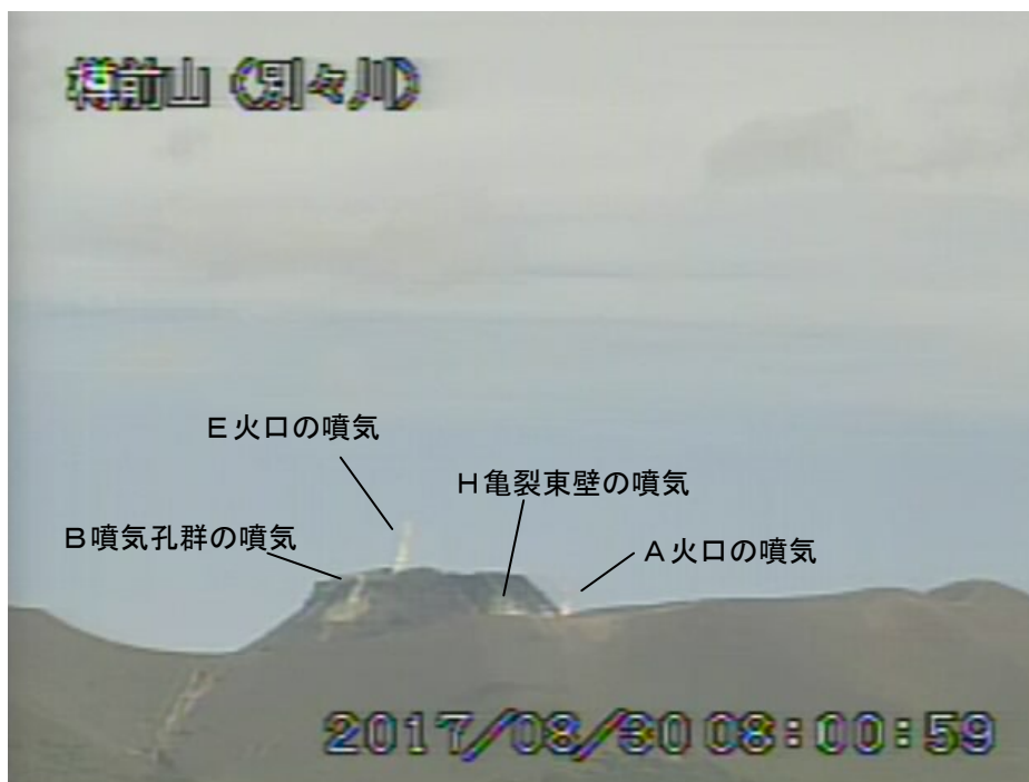
図 2 樽前山 南側から見た山頂部の状況 (8月30日、別々川監視カメラによる)
