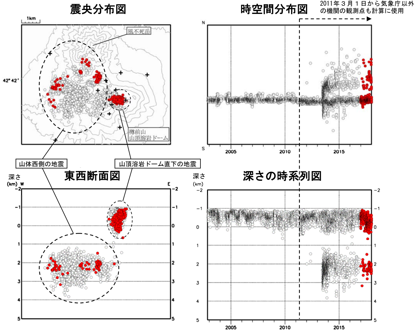
図 9 樽前山 火山性地震の震源分布 (2002年11月～2017年12月)
