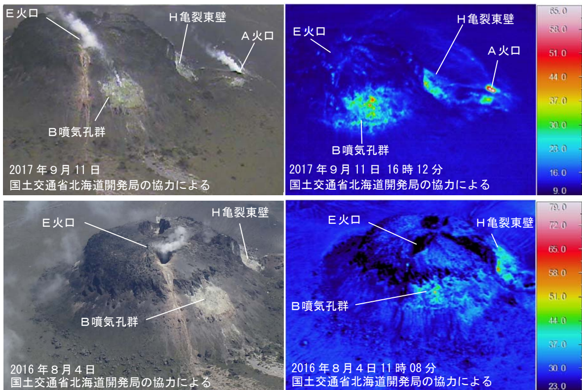
図 5 樽前山 赤外熱映像装置による山頂溶岩ドーム周辺の地表面温度分布 上：南西側上空（図3の③）から撮影 下：南西側上空（図3の④）から撮影 ・山頂溶岩ドームの噴気や地表面温度分布の状況に変化は認められませんでした
