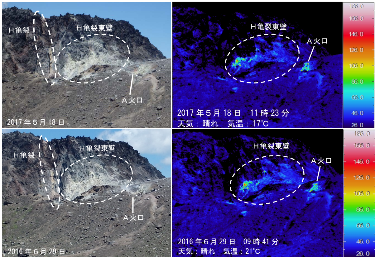
図 6 樽前山 赤外熱映像装置によるA火口、H亀裂及び周辺の地表面温度分布 南東側（図3の⑤）から撮影
