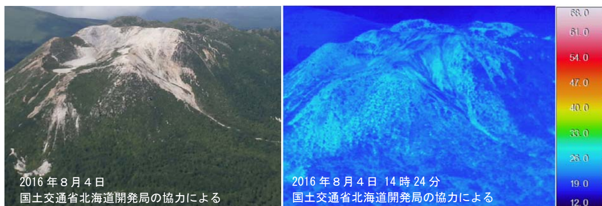
図 4 ニセコ 赤外熱映像装置によるイワオヌプリ山頂部の地表面温度分布 図 1 中の③から撮影
