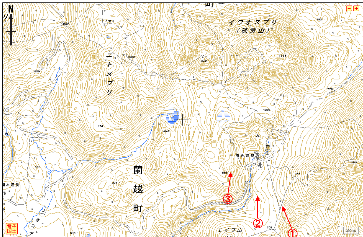
図 1 ニセコ 周辺図と赤外熱映像及び写真の撮影方向（矢印）
